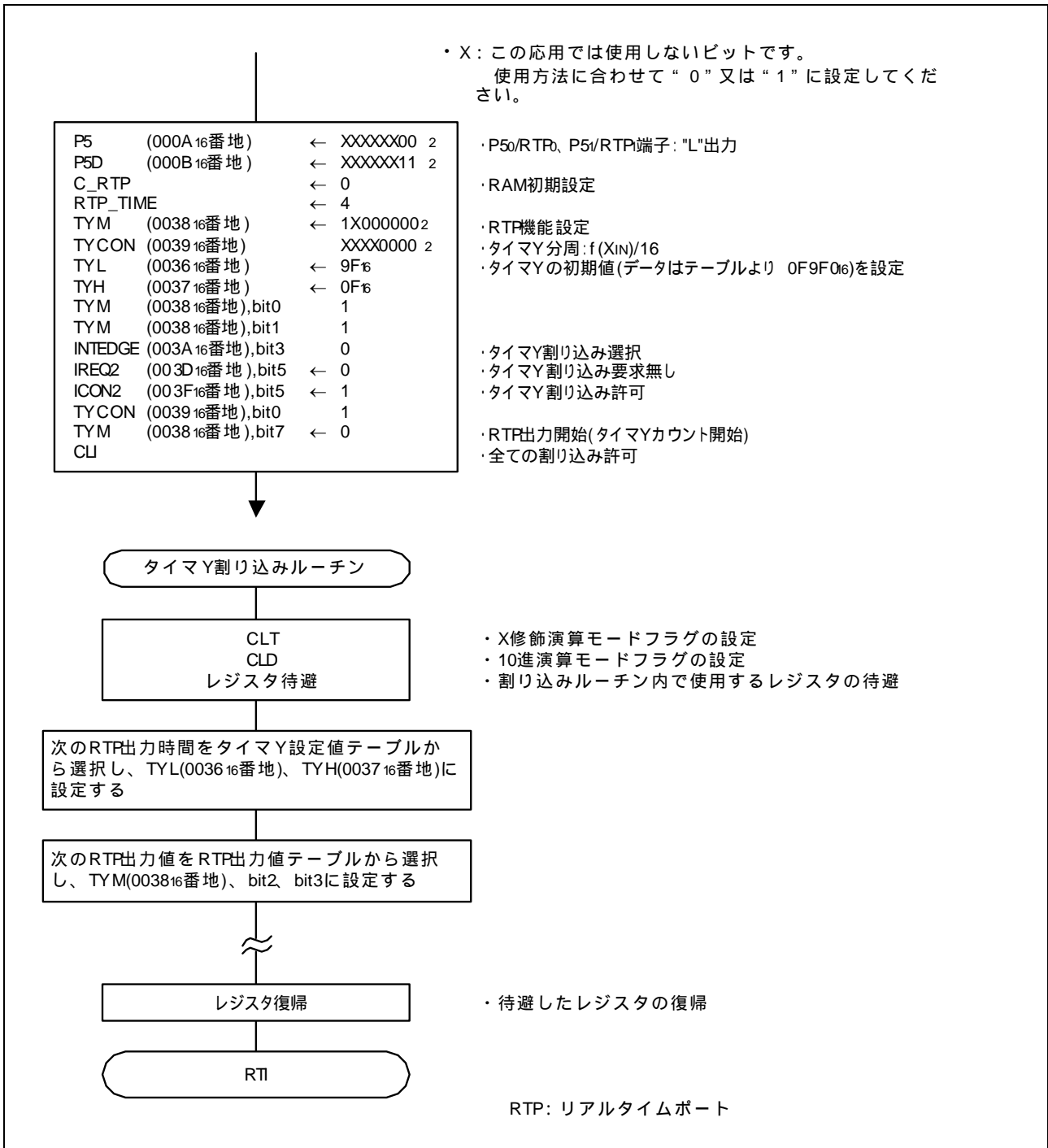
図 3.4 制御手順
