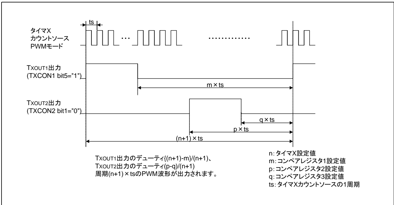
図 3.2 PWM(TXOUT1/TXOUT2) 出力波形
