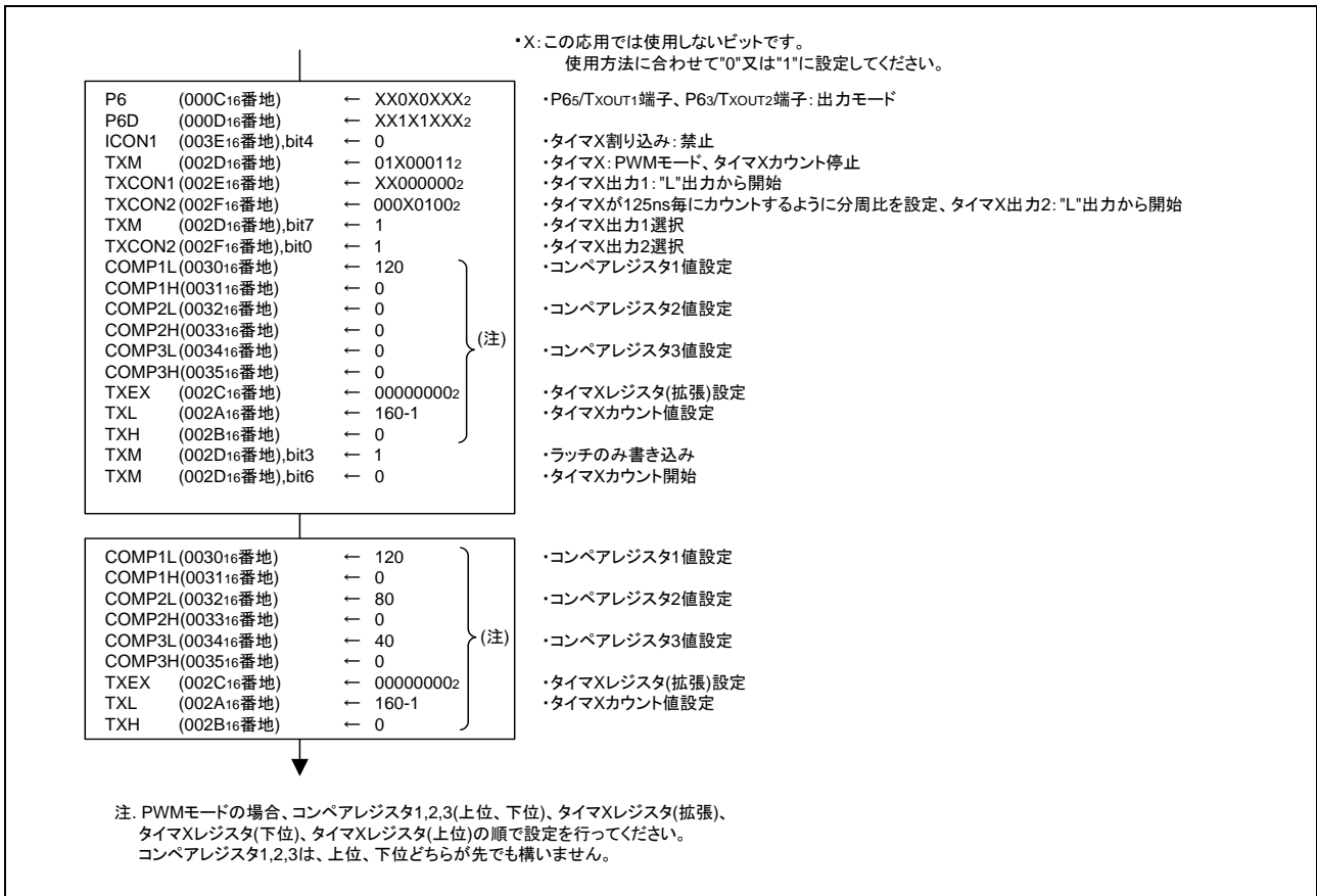
図 3.5 制御手順
