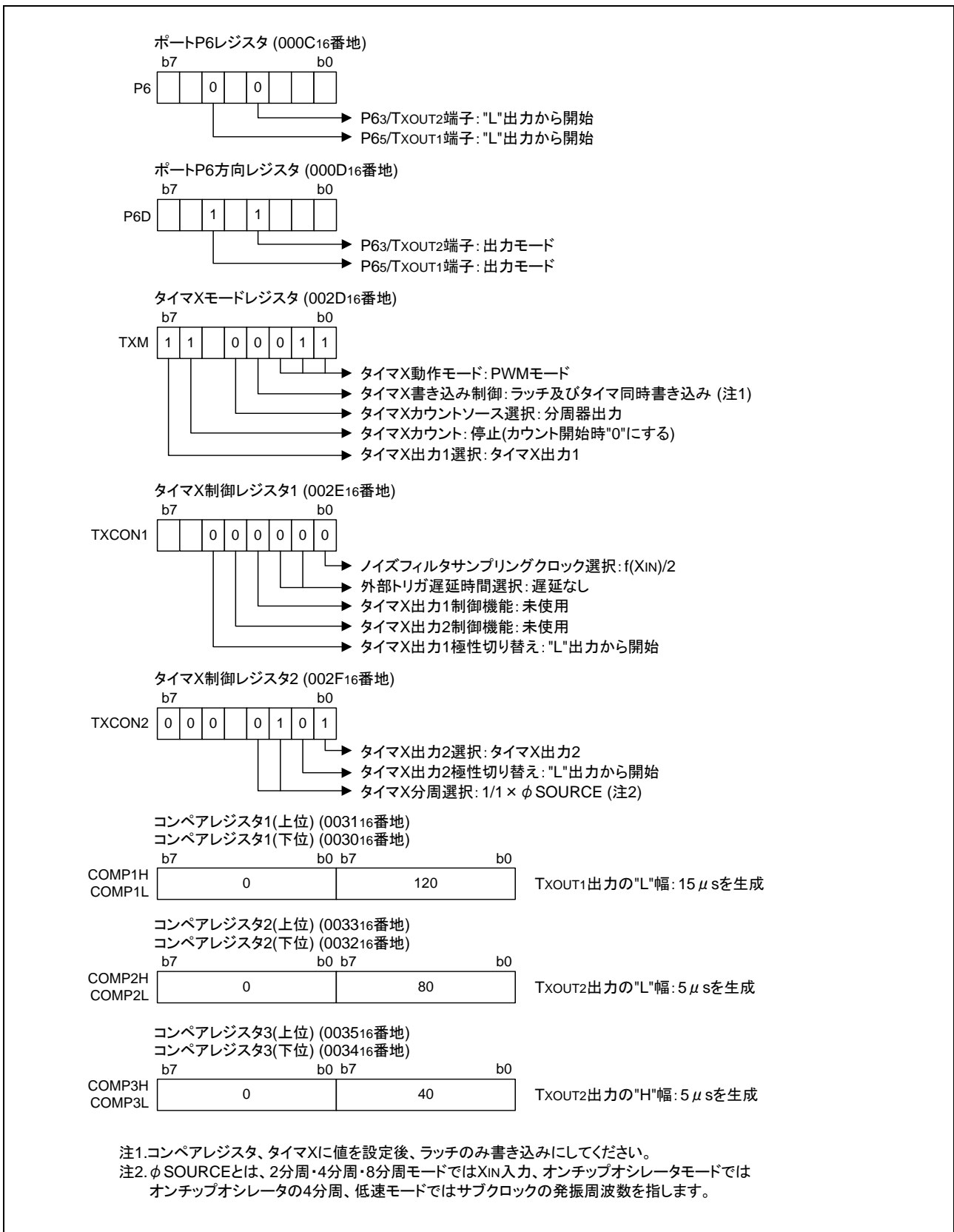
図 3.3 関連レジスタの設定 (1)
