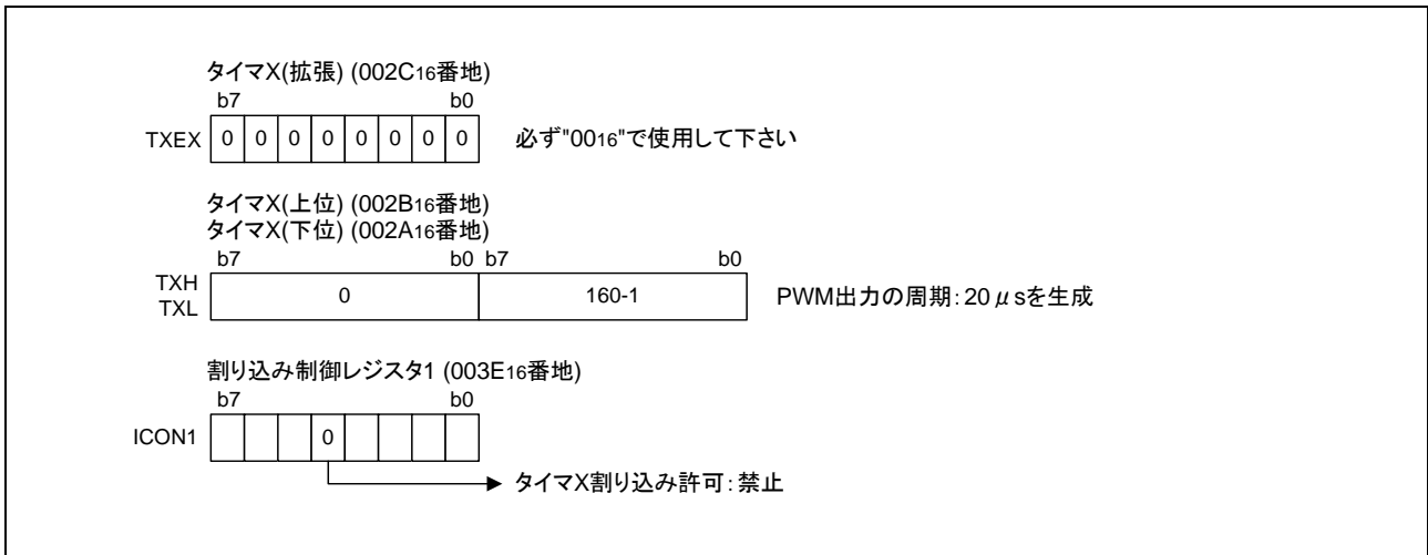
図 3.4 関連レジスタの設定 (2)
