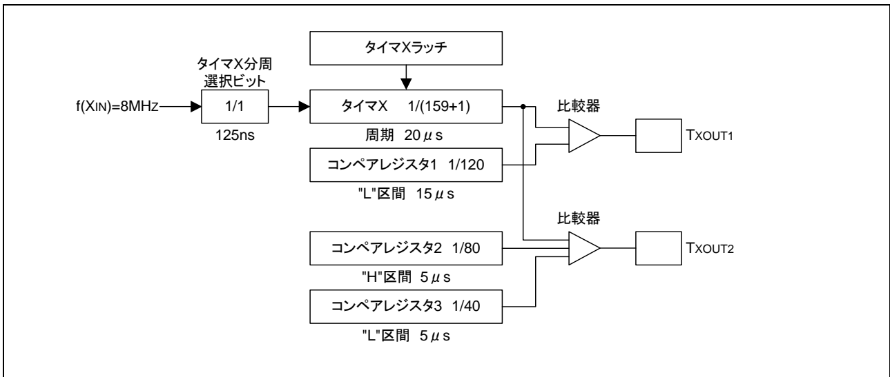
図 3.1 タイマの接続と分周比
