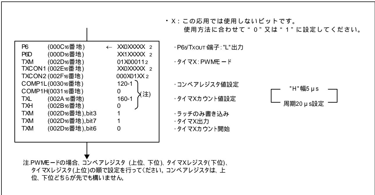
図 3.3 制御手順
