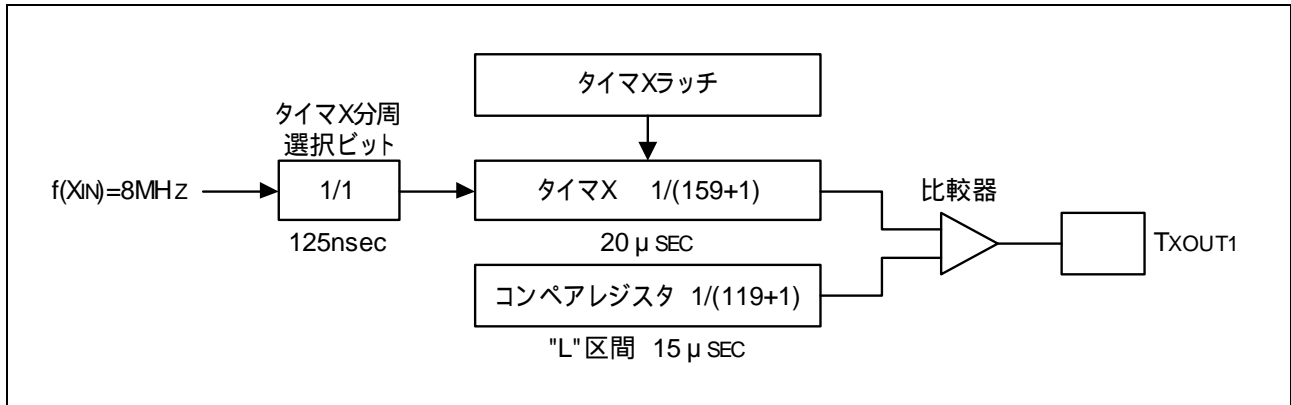
図 3.1 タイマの接続と分周比
