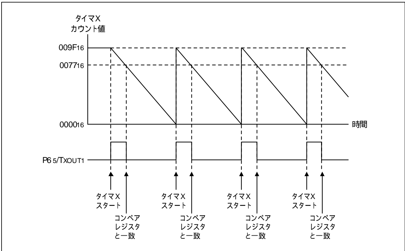
図 3.4 PWM(TXOUT) 出力波形
