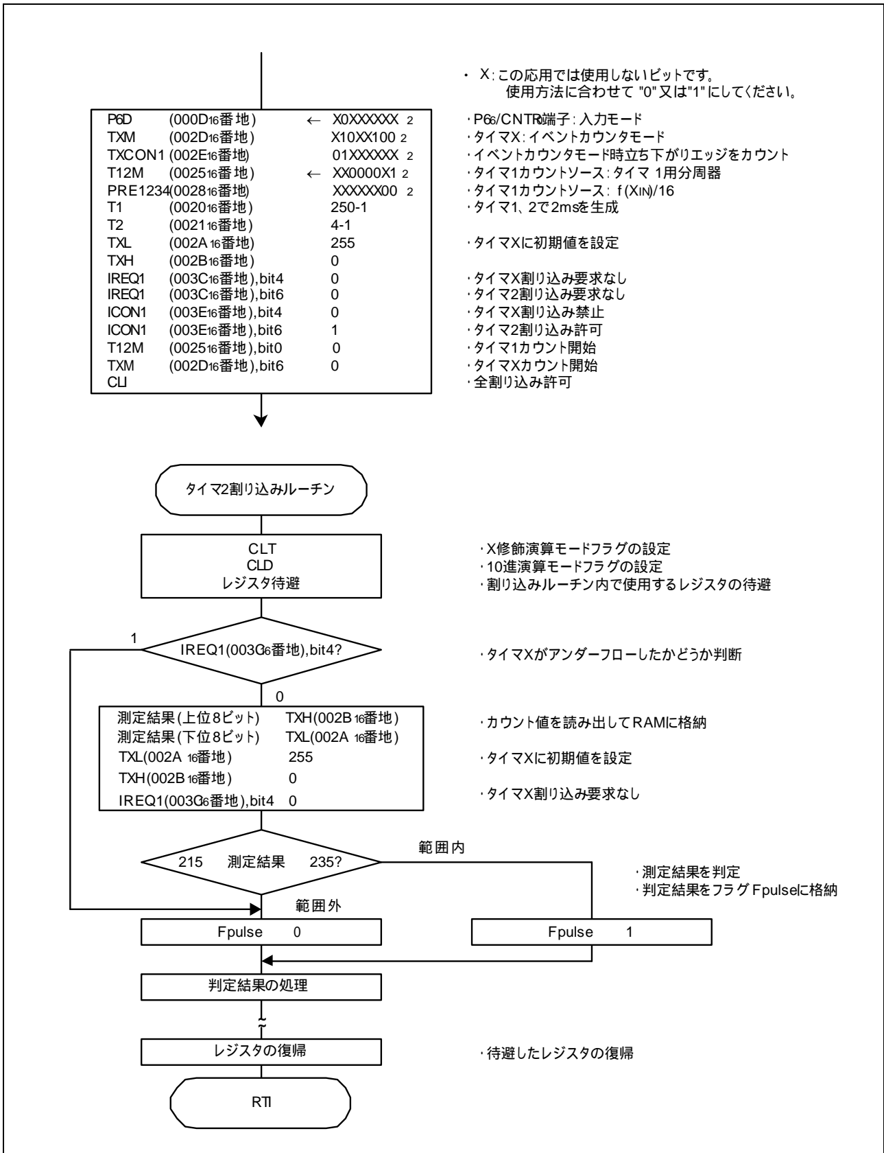
図 3.4 制御手順
