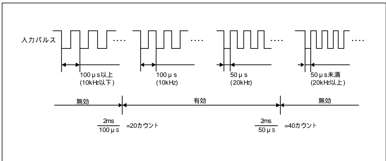
図 3.1 入力パルス有効又は無効の判定方法
