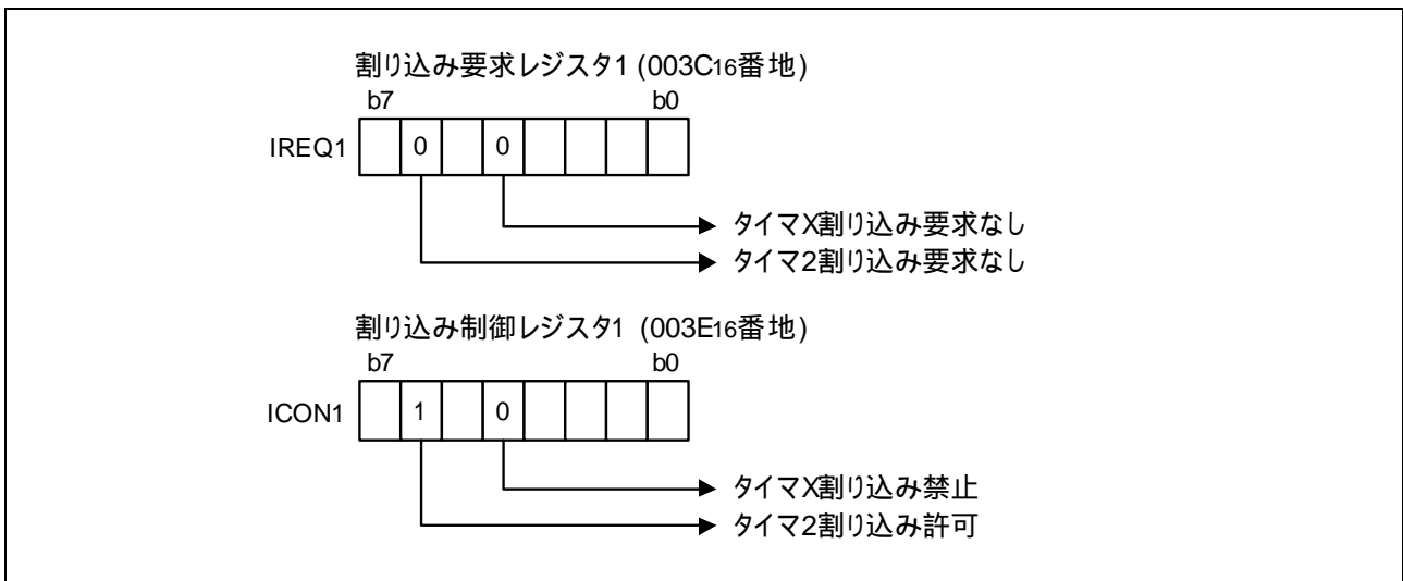
図 3.3 関連レジスタの設定 (2)
