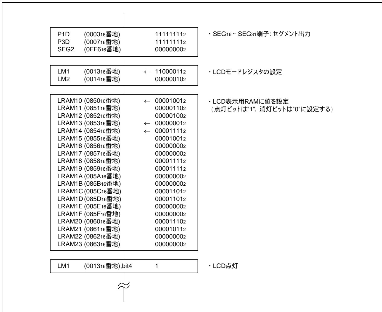
図 3.6 制御手順
