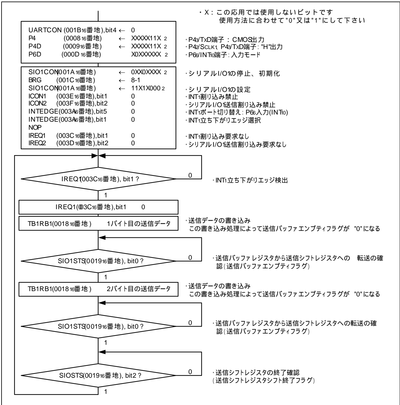
図 3.5 送信側の制御手順
