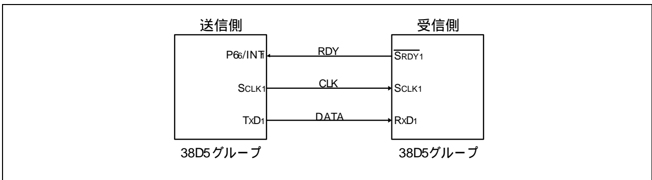
図 3.1 接続図
