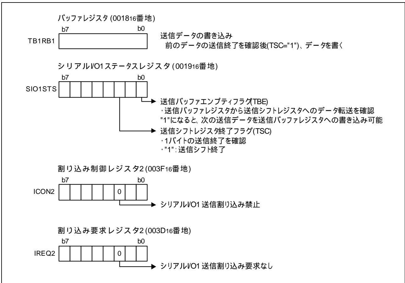
図 3.3 送信側関連レジスタの設定
