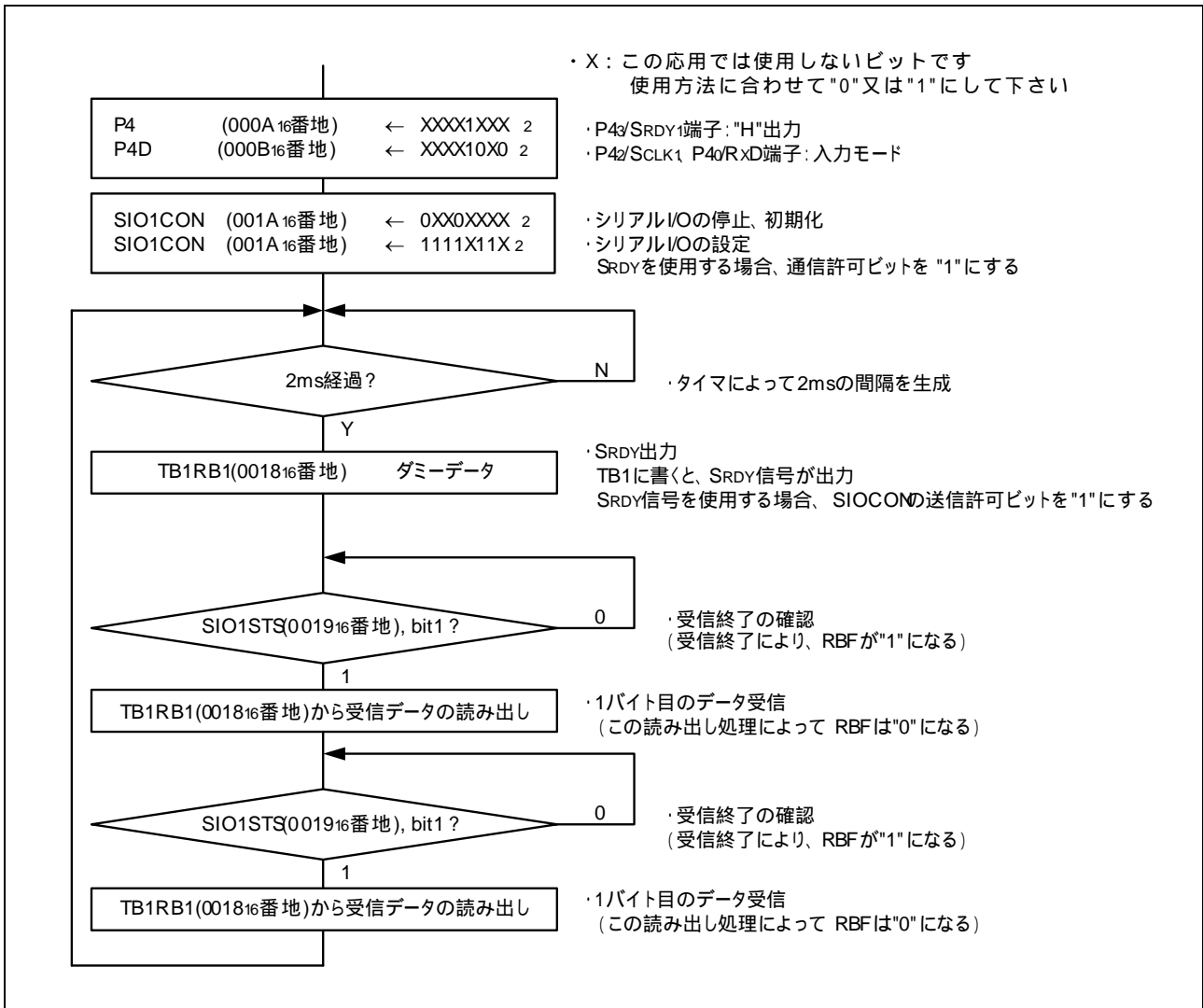
図 3.6 受信側の制御手順
