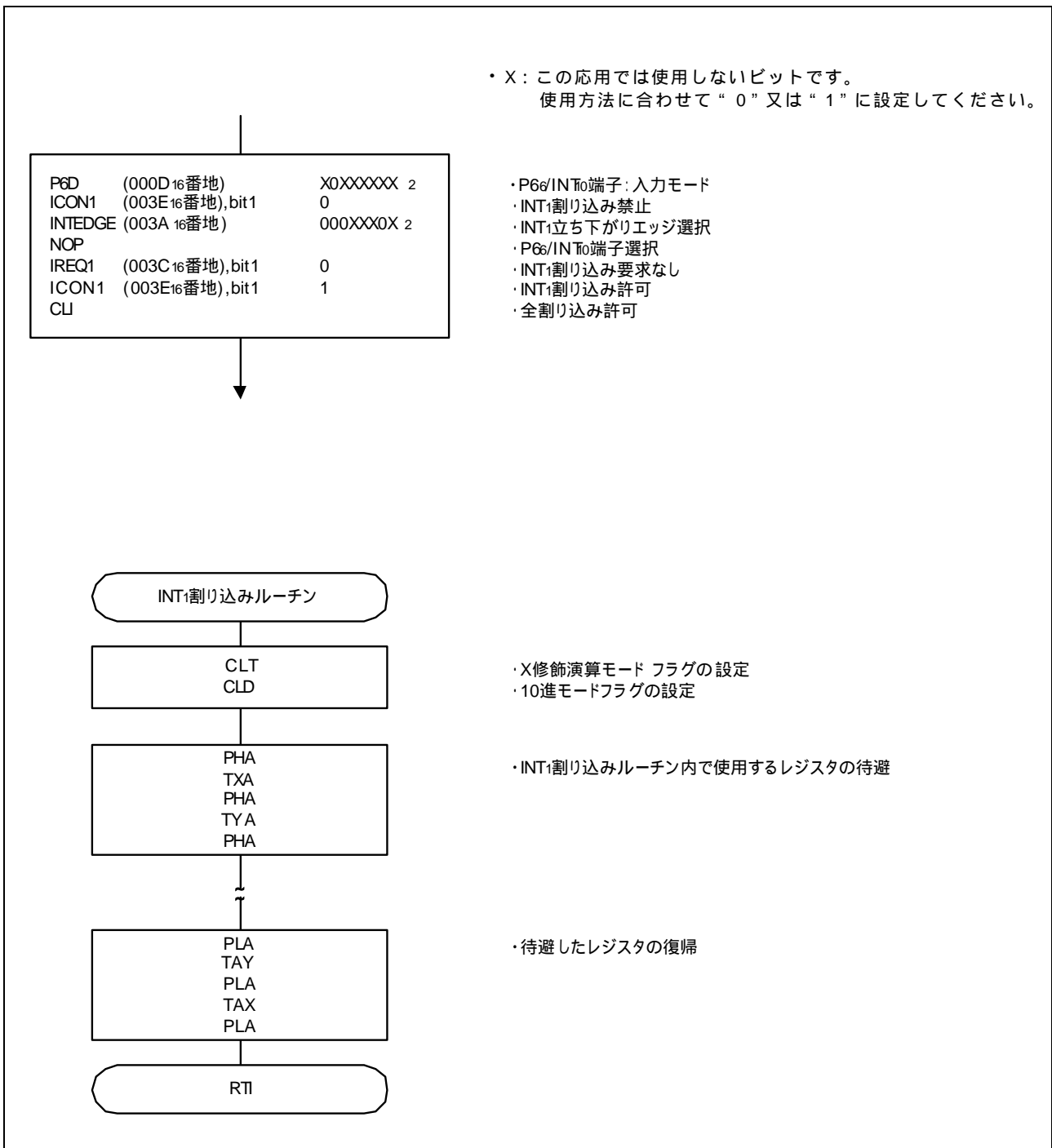
図 3.3 制御手順
