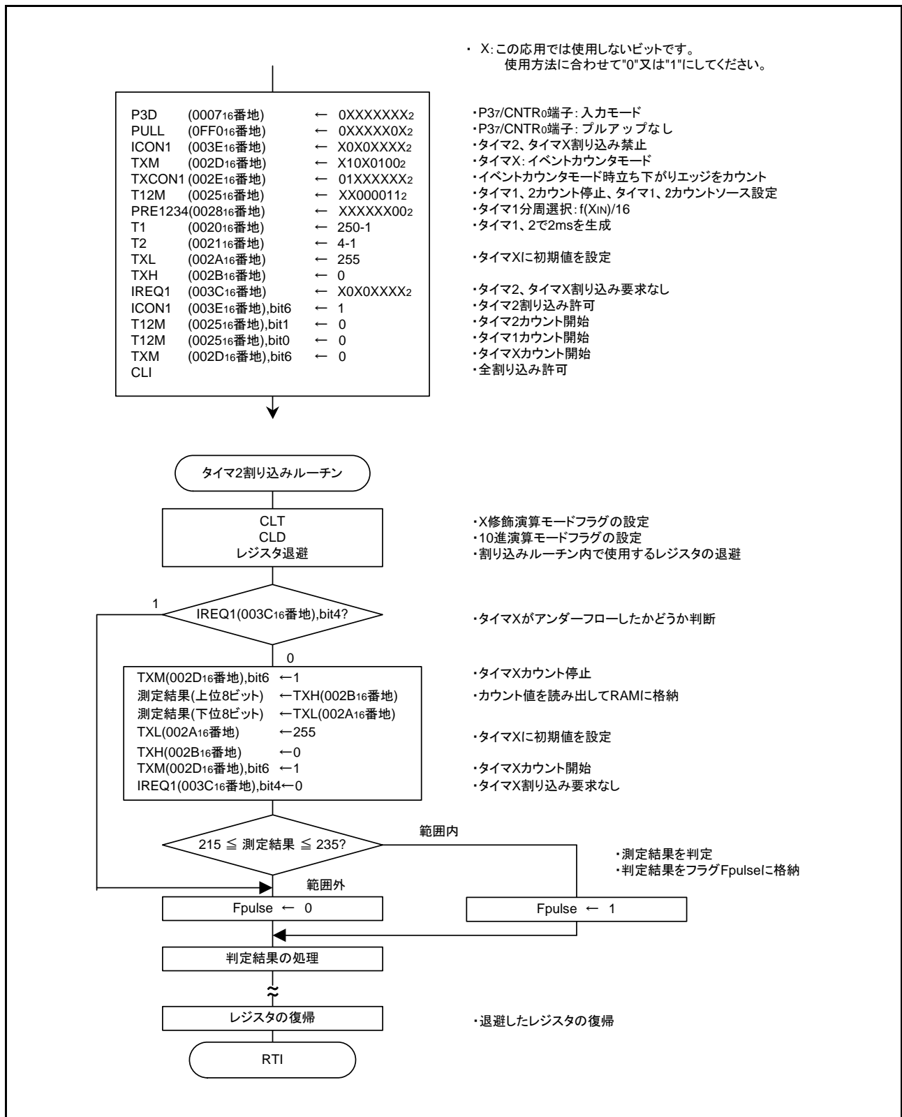
図 3.4 制御手順
