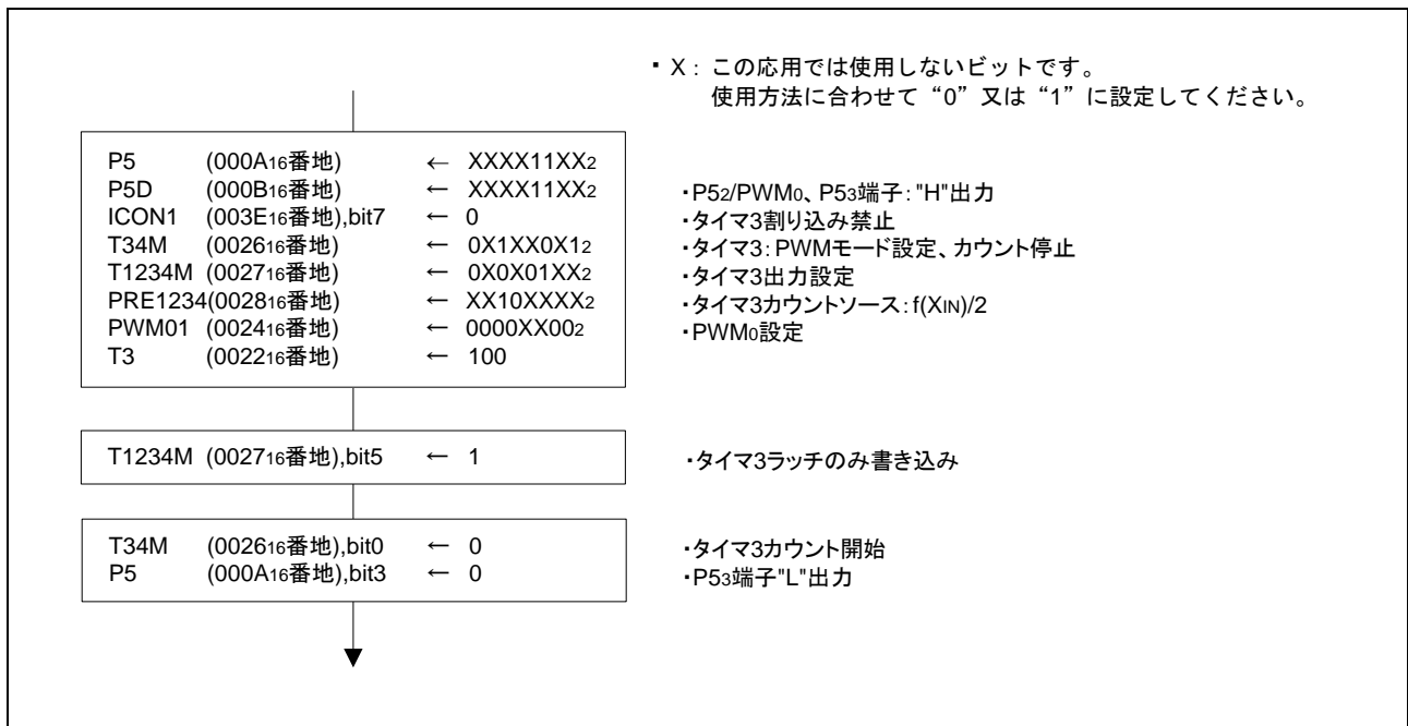
図 3.4 制御手順
