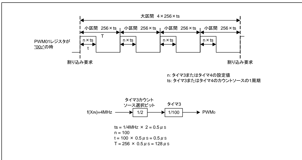
図 3.2 PWM0 及び PWM1 の出力波形図
