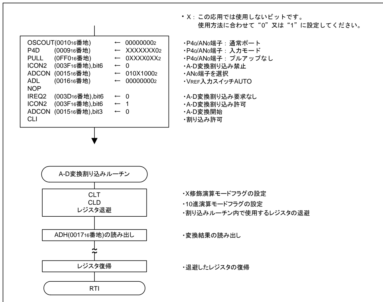
図 3.3 制御手順
