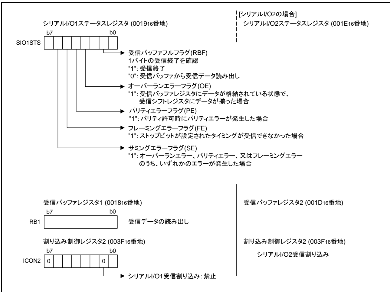
図 3.5 受信側関連レジスタの設定 (2)
