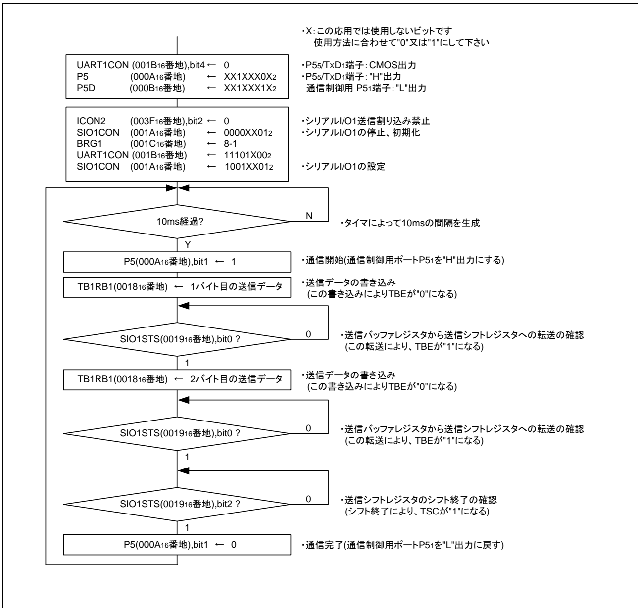
図 3.6 送信側の制御手順
