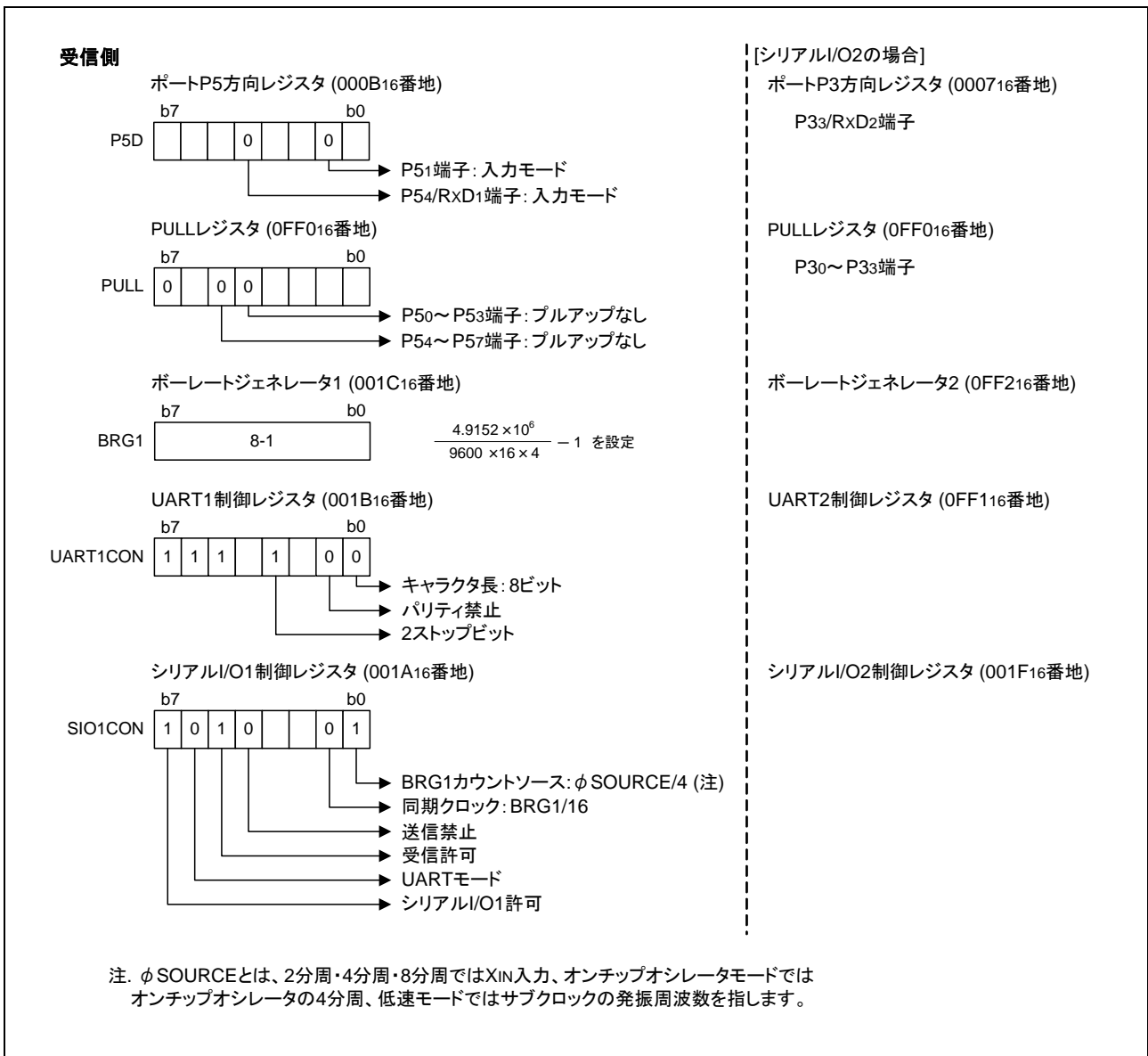
図 3.4 受信側関連レジスタの設定 (1)
