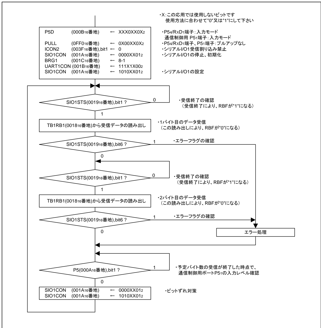
図 3.7 受信側の制御手順
