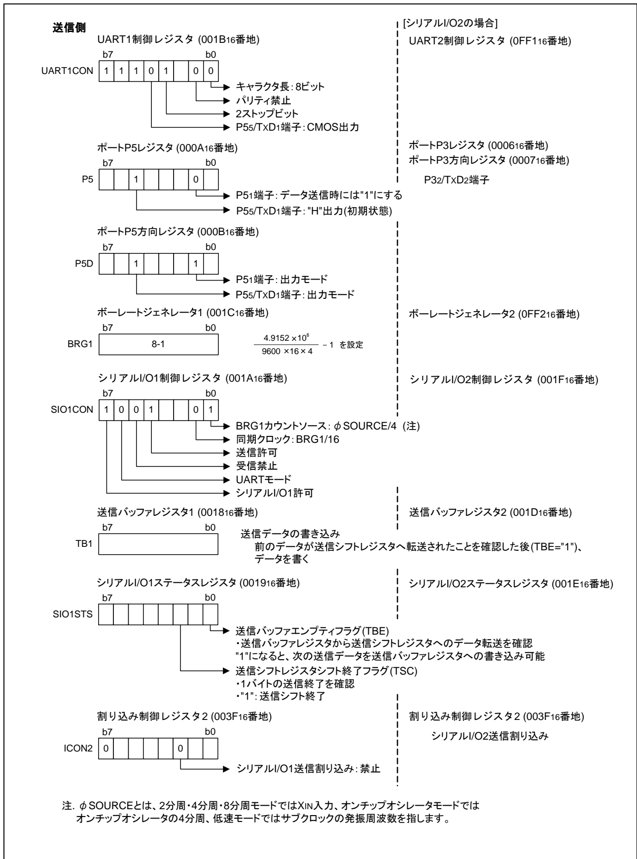
図 3.3 送信側関連レジスタの設定
