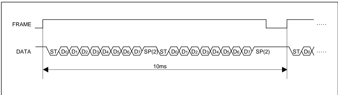
図 3.2 タイミング図
