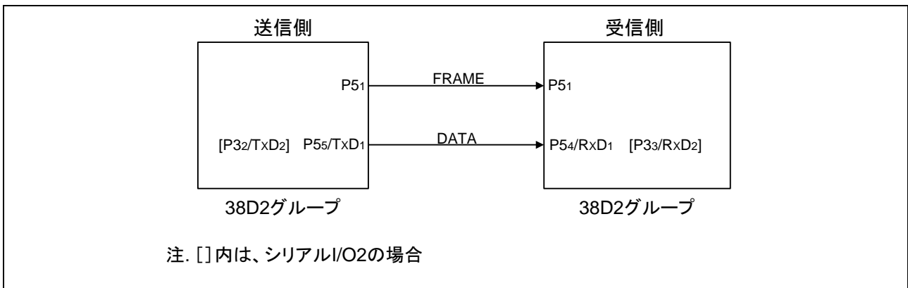
図 3.1 接続図
