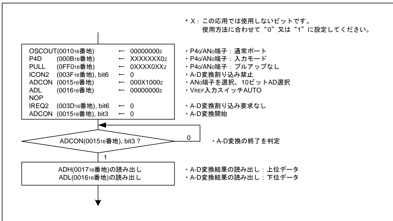
図 3.3 制御手順
