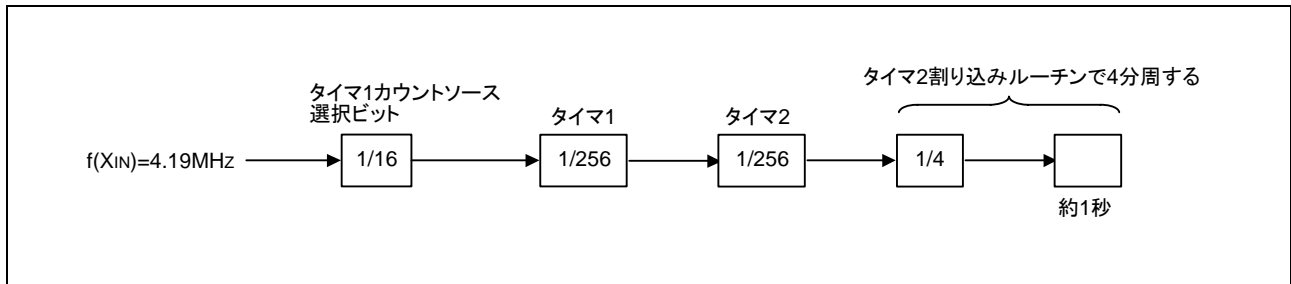
図 3.1 タイマの接続と分周比
