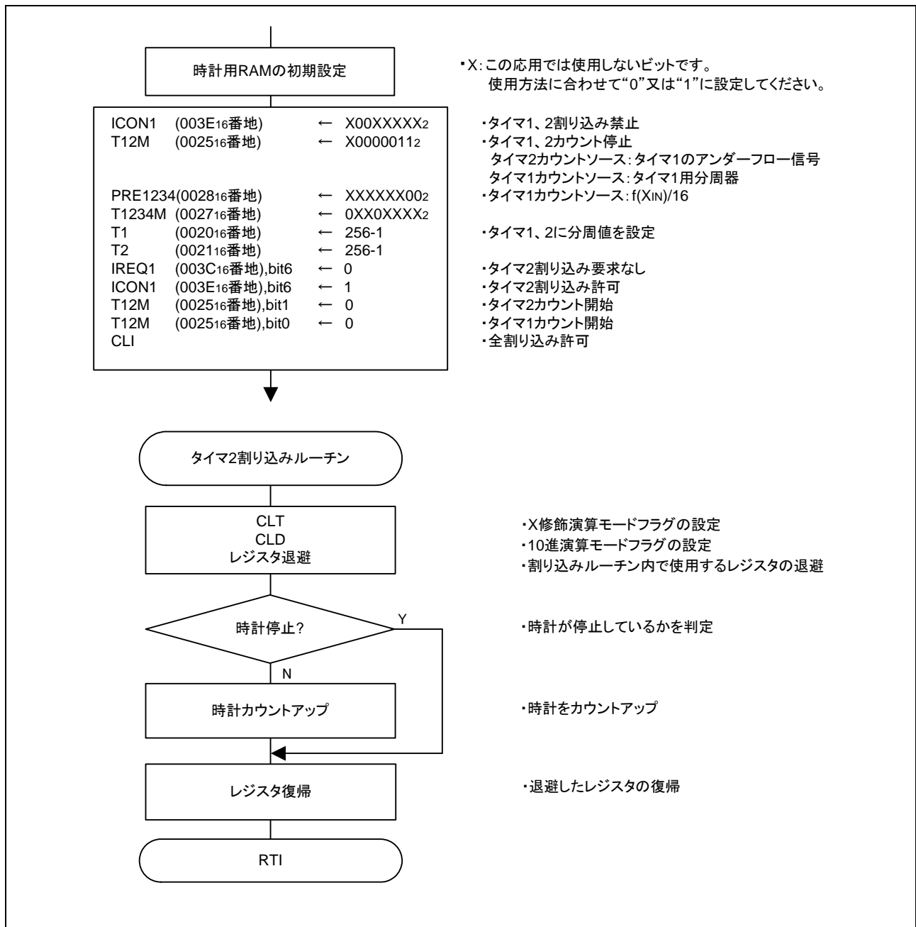
図 3.3 制御手順
