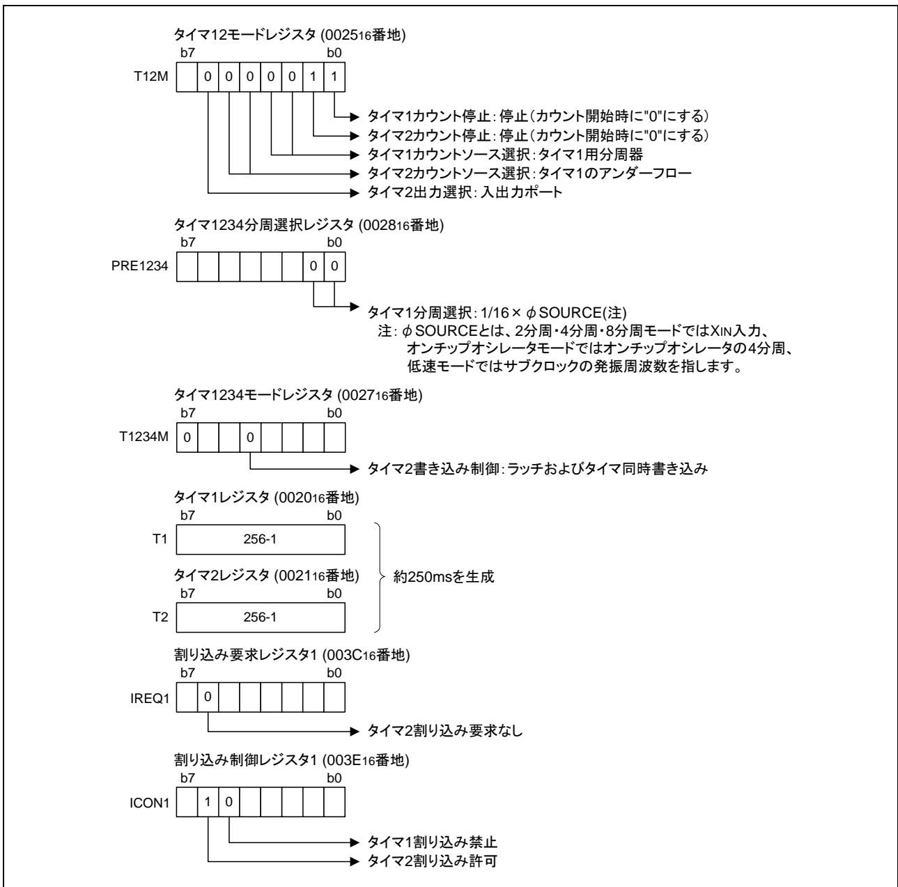
図 3.2 関連レジスタの設定
