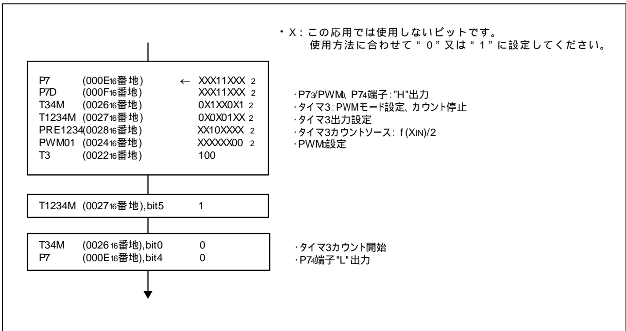
図 3.4 制御手順
