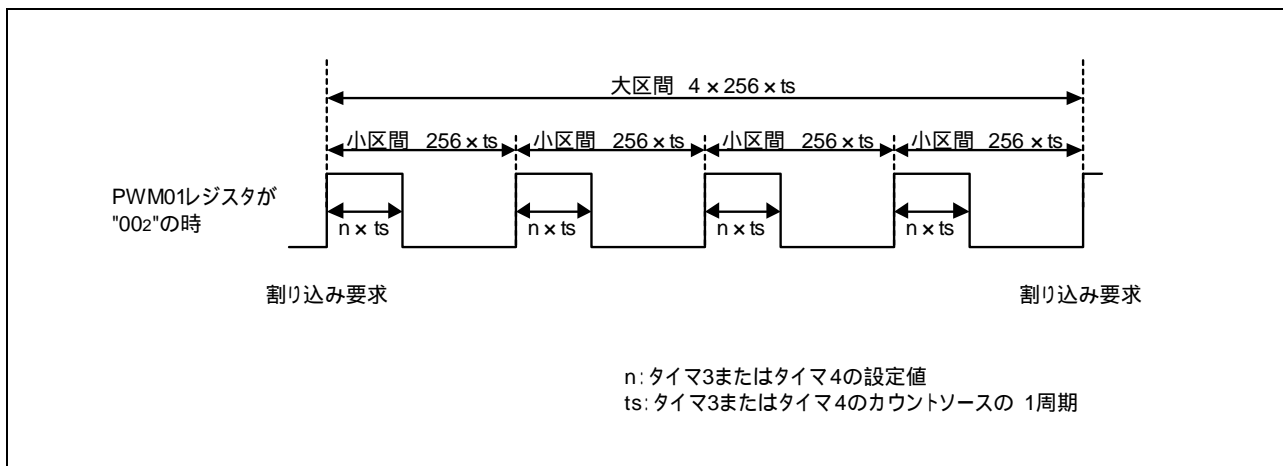
図 3.2 PWM0 及び PWM1 の出力波形図
