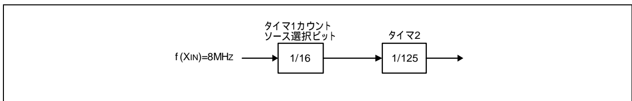
図 3.2 タイマの接続と分周比
