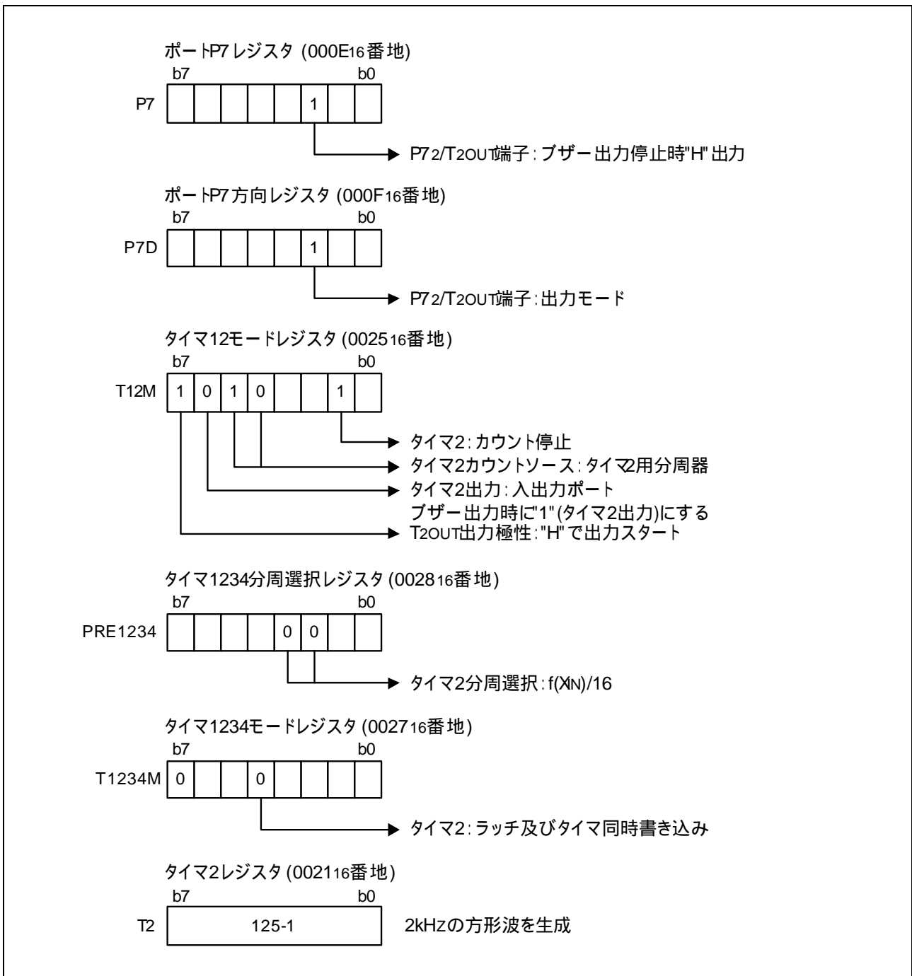
図 3.3 関連レジスタの設定
