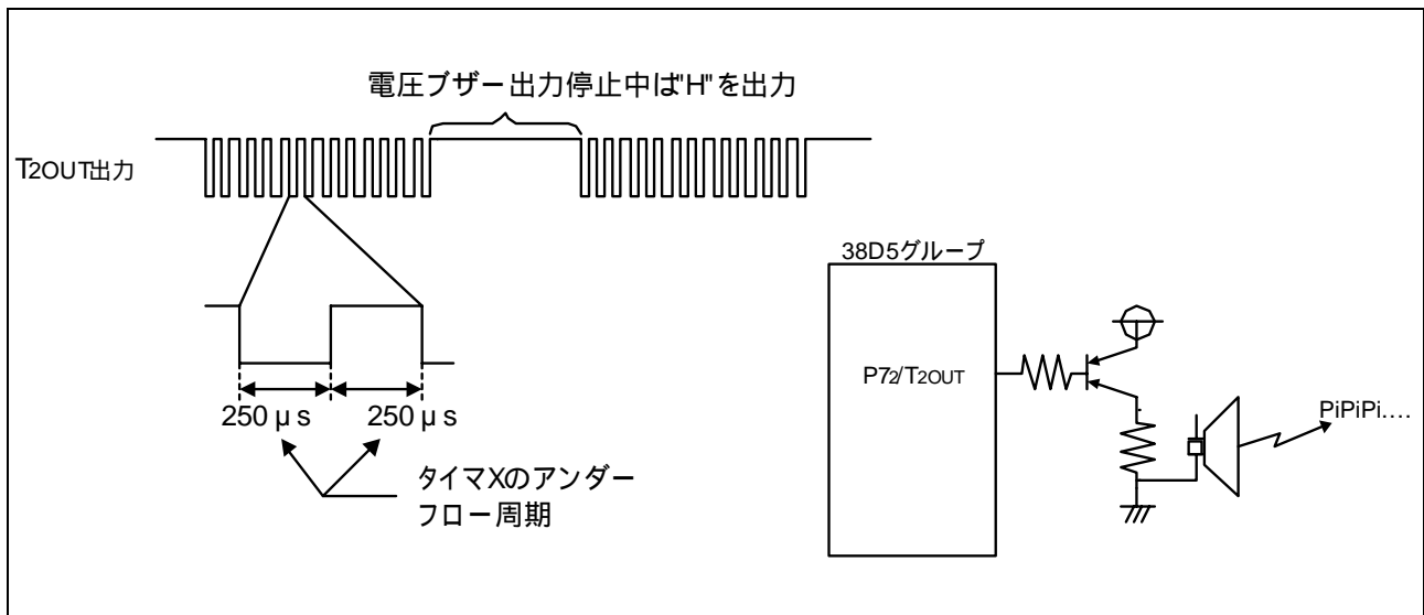
図 3.1 出力波形図及び周辺回路例
