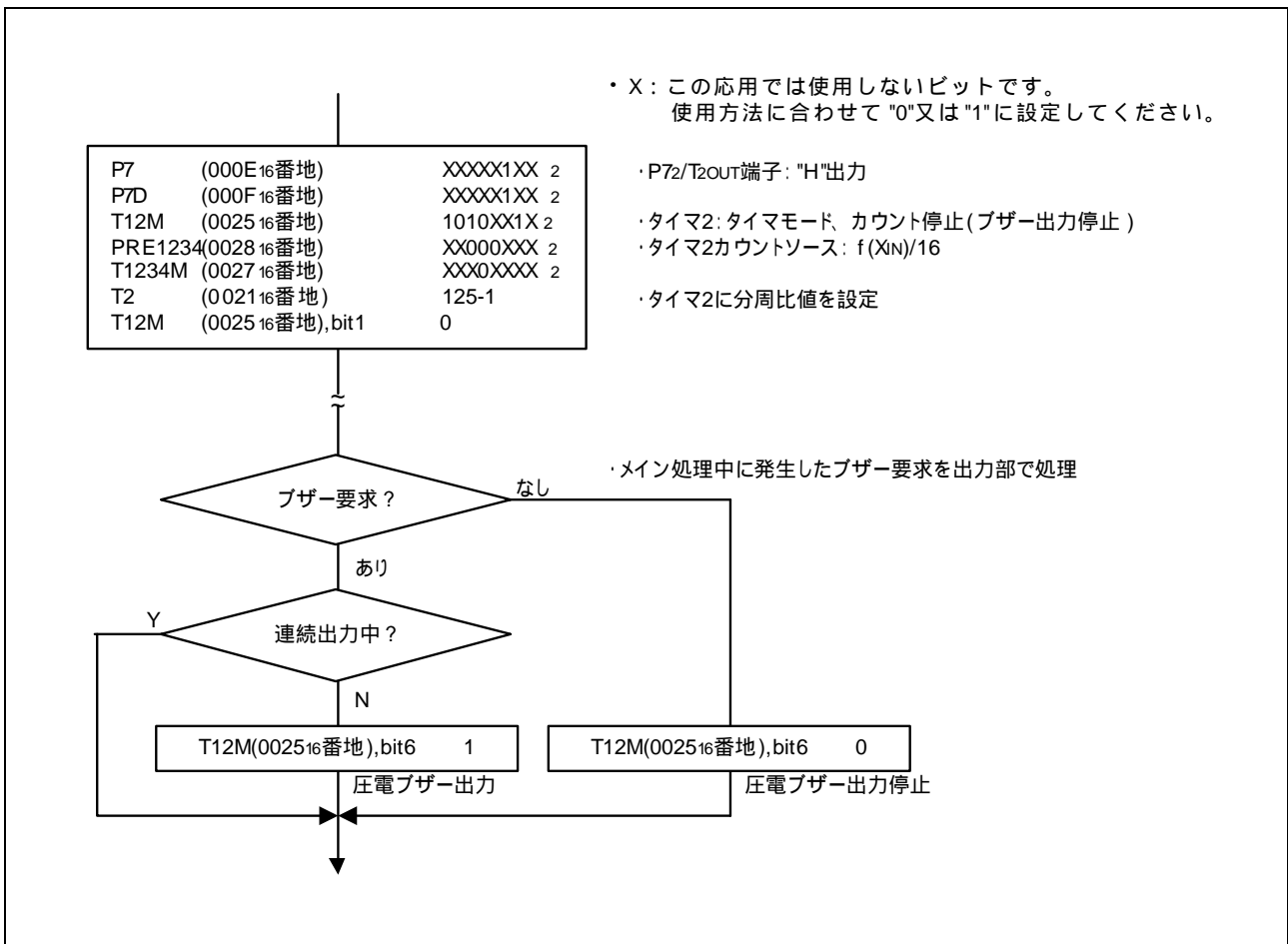
図 3.4 制御手順
