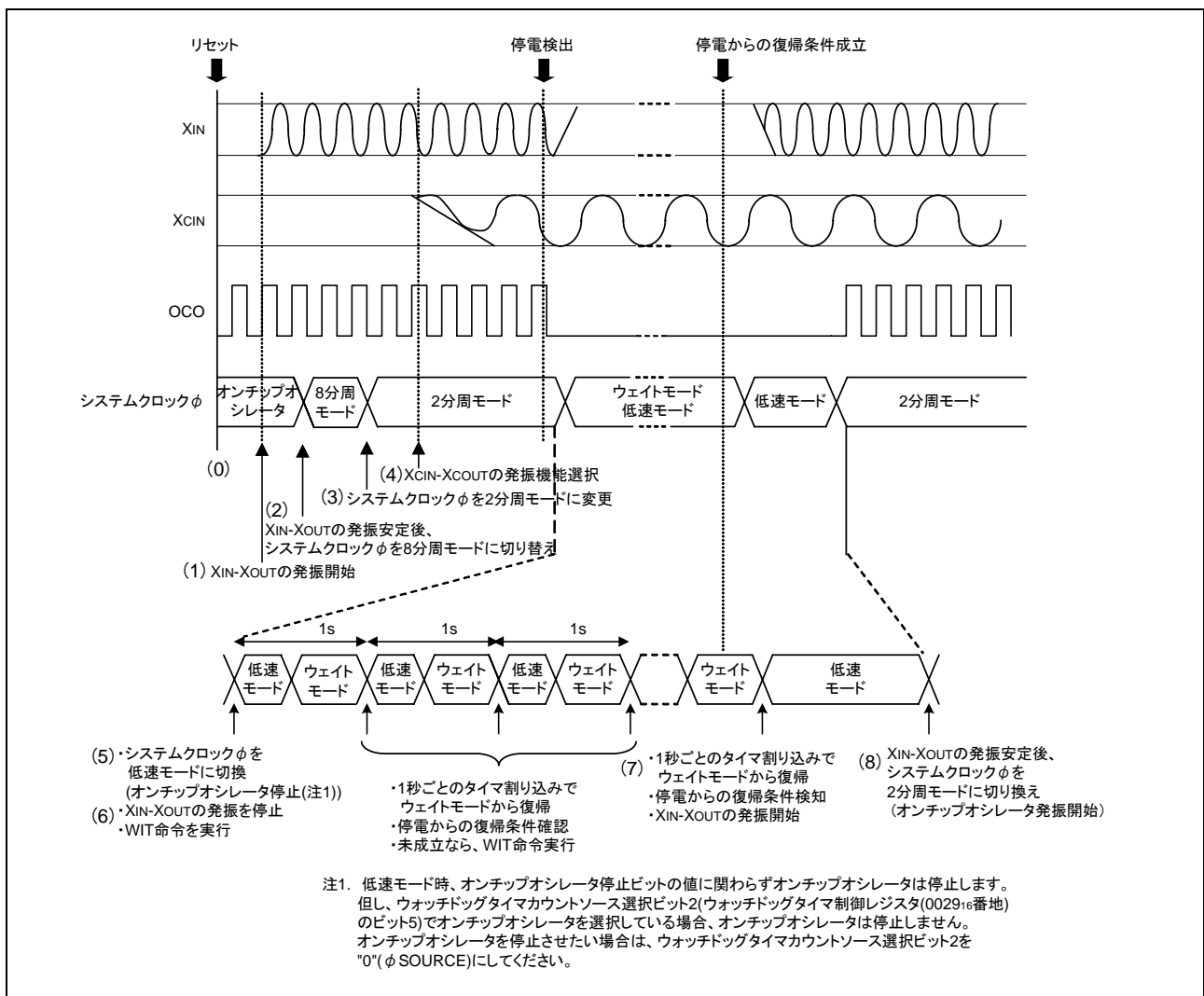
図 3.1 停電時のシステムクロック \phi のモード移行例 ( OSCSEL="L" 時 )
