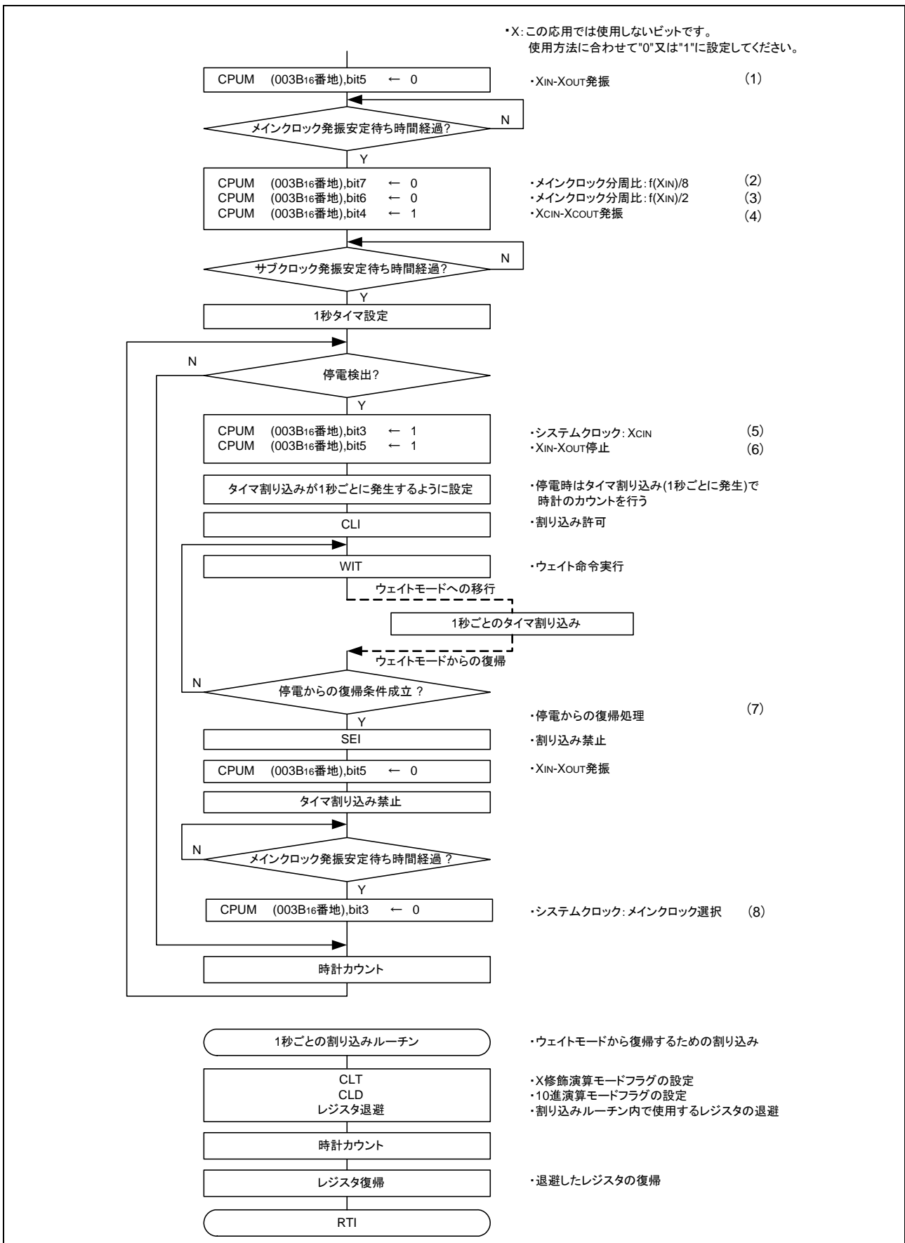
図 3.3 制御手順
