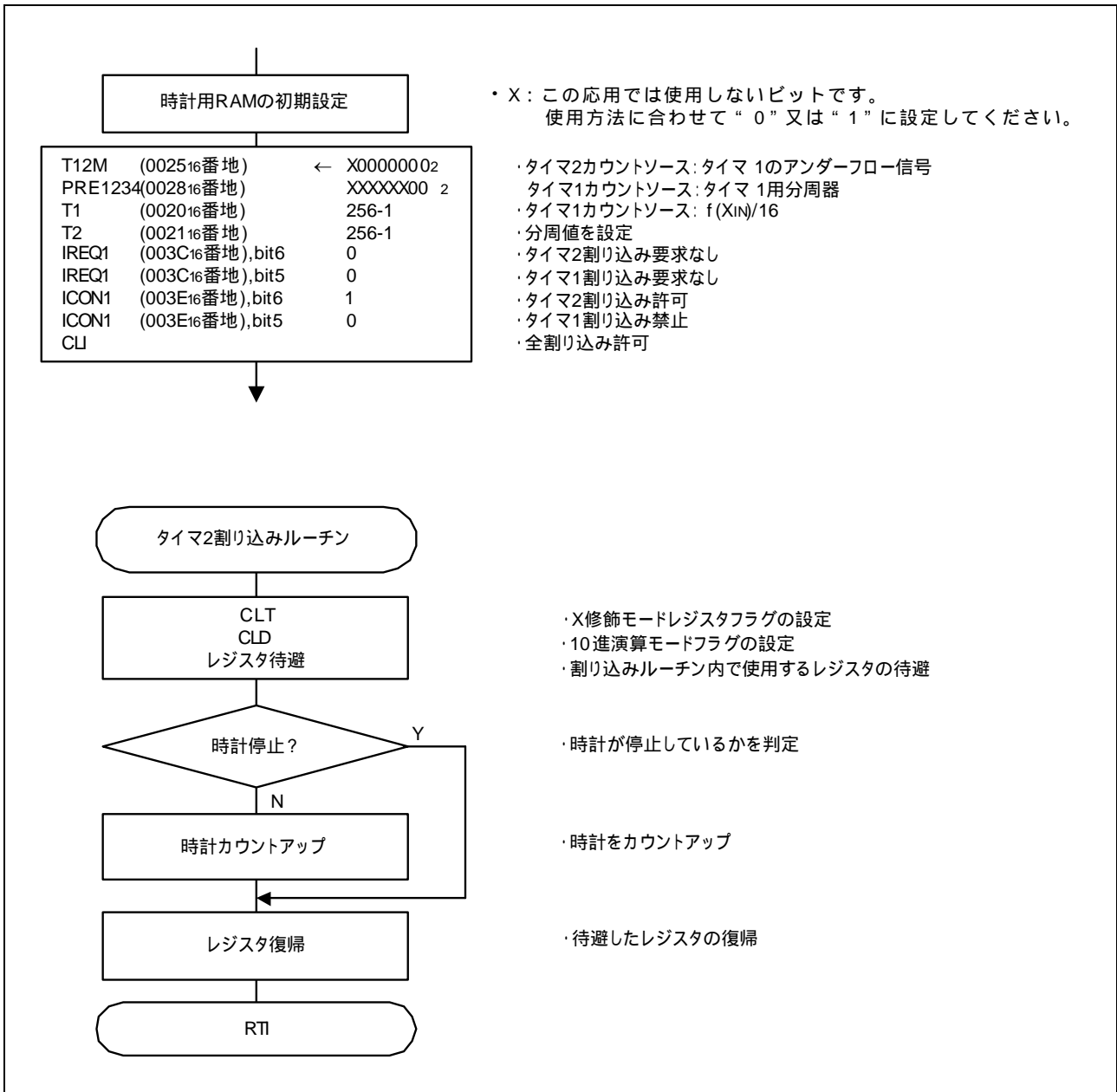
図 3.3 制御手順
