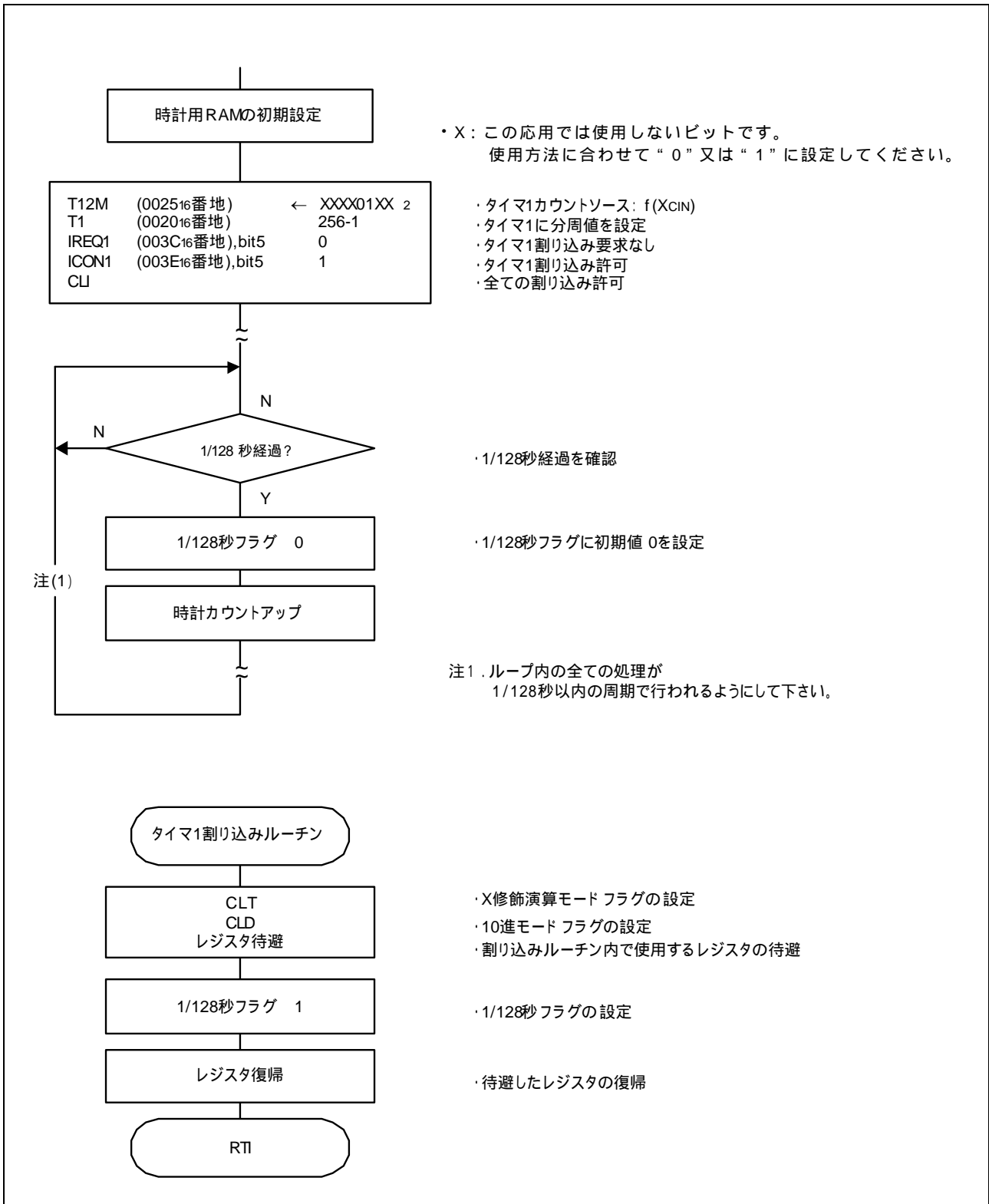
図 3.3 制御手順
