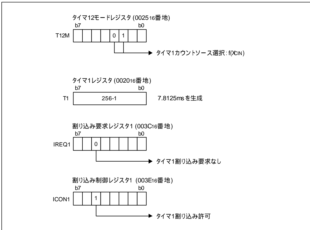
図 3.2 関連レジスタの設定
