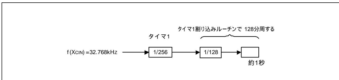
図 3.1 タイマの接続と分周比
