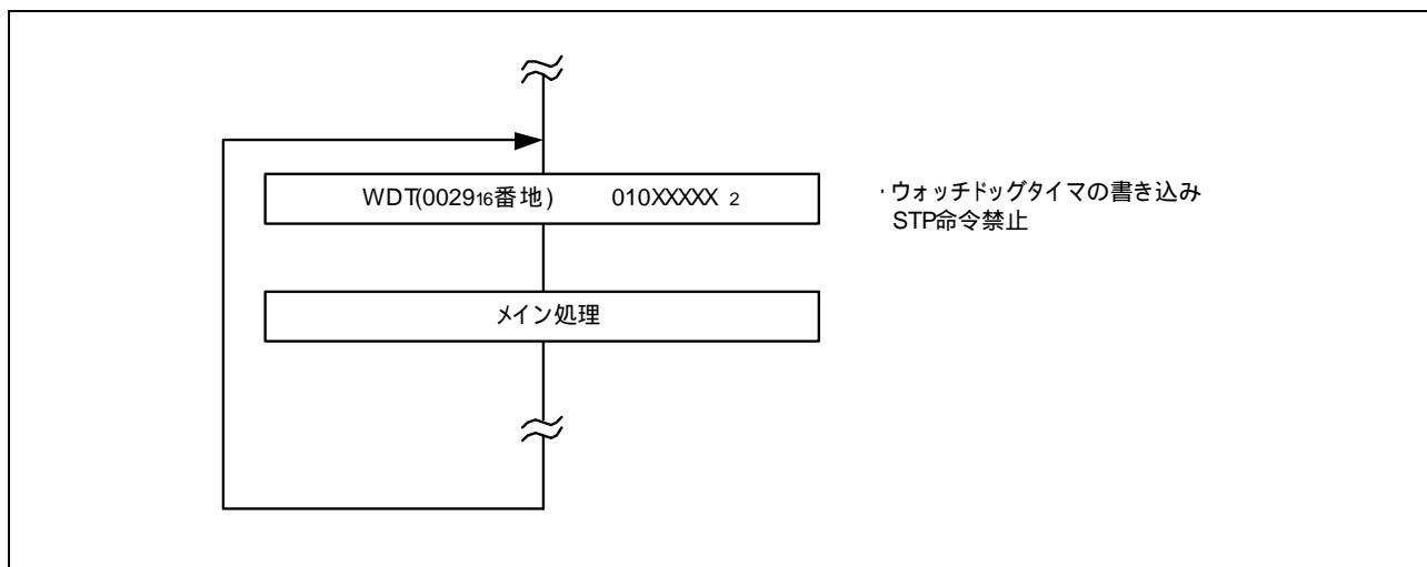
図 3.3 制御手順
