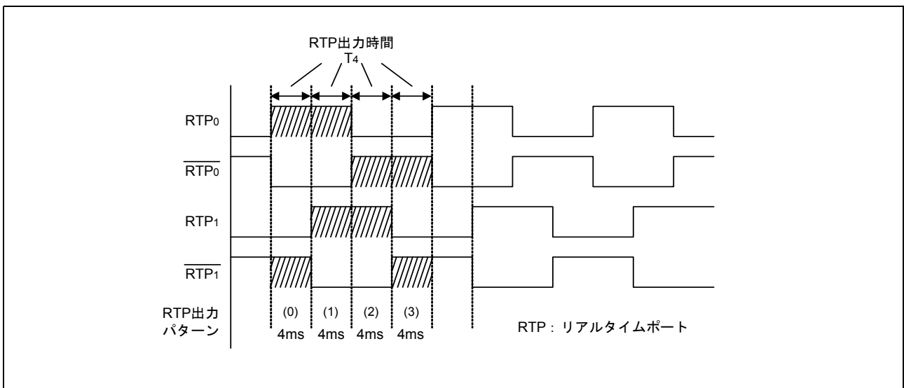
図 3.2 RTP 出力例
