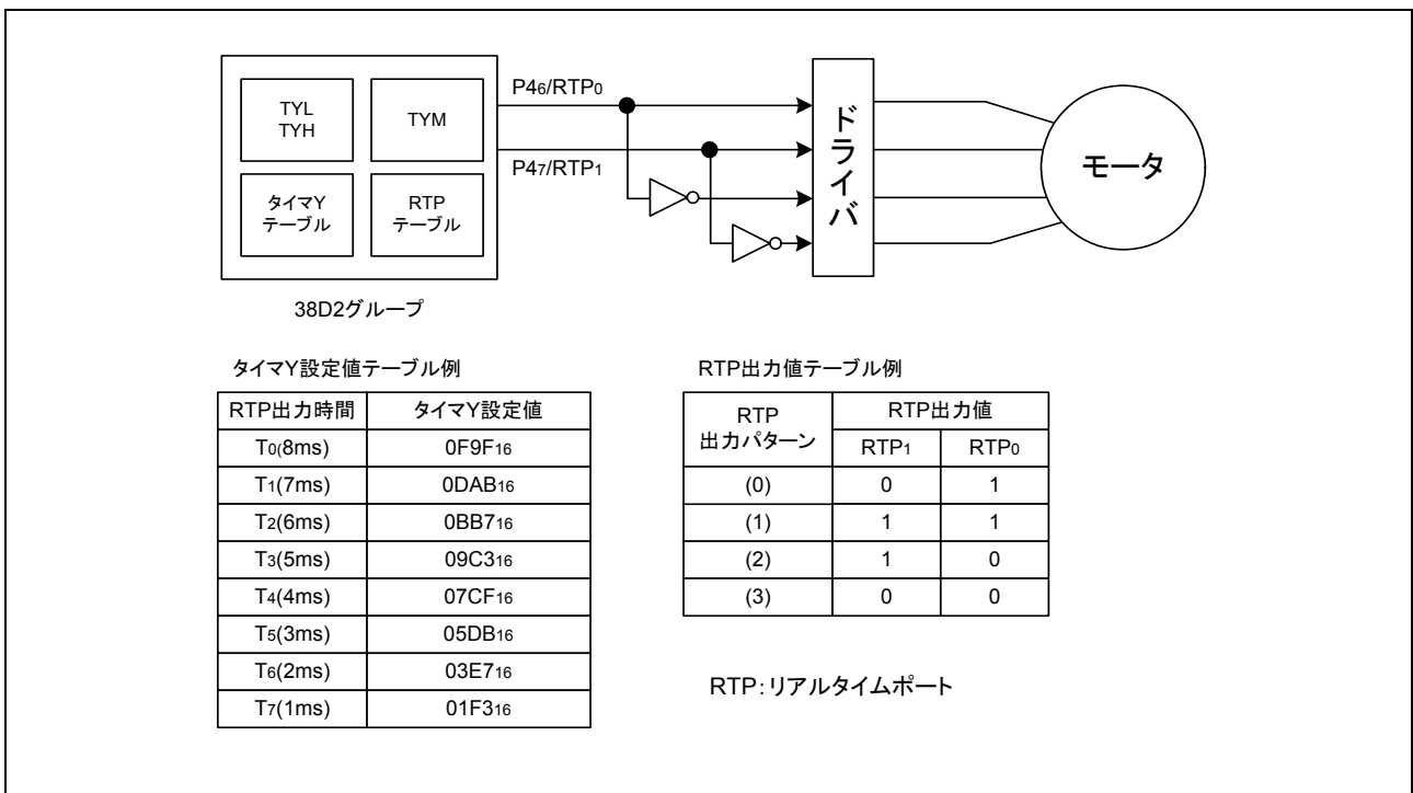
図 3.1 接続図、タイマ Y 設定値テーブル例及び RTP 出力値テーブル例
