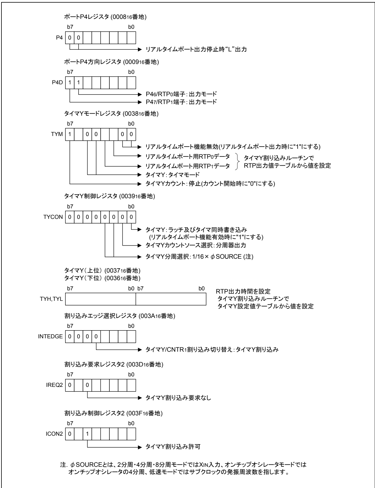
図 3.3 関連レジスタの設定
