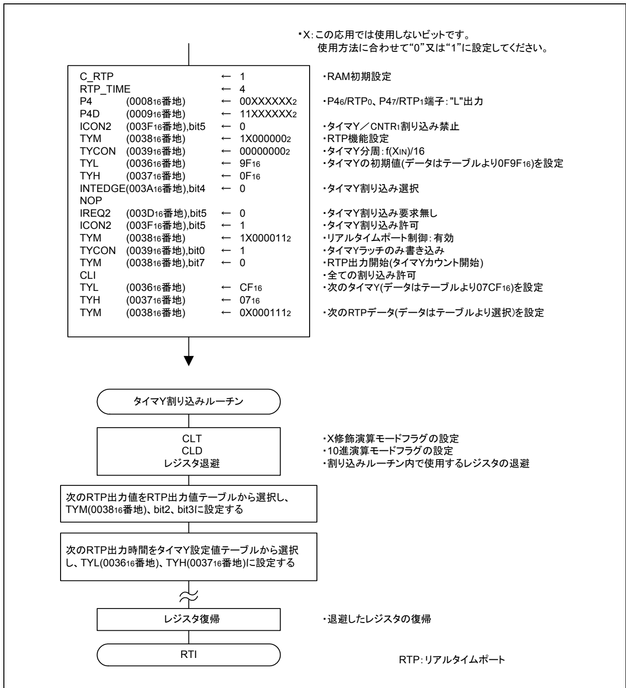
図 3.4 制御手順
