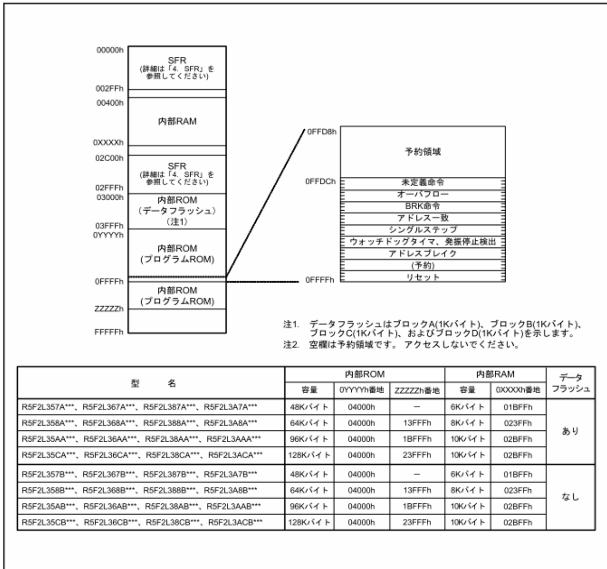
図3.5 R8C/L36Aグループのメモリ配置図
