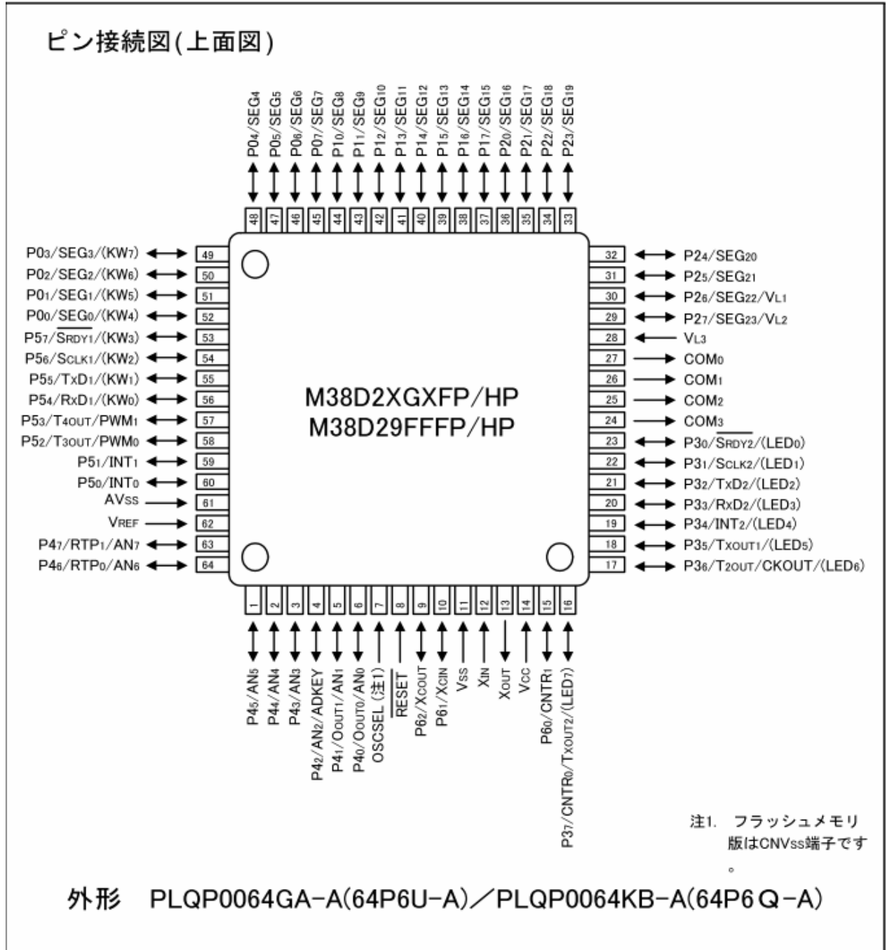
図3.1 38D2グループピン配置図(QFP)
