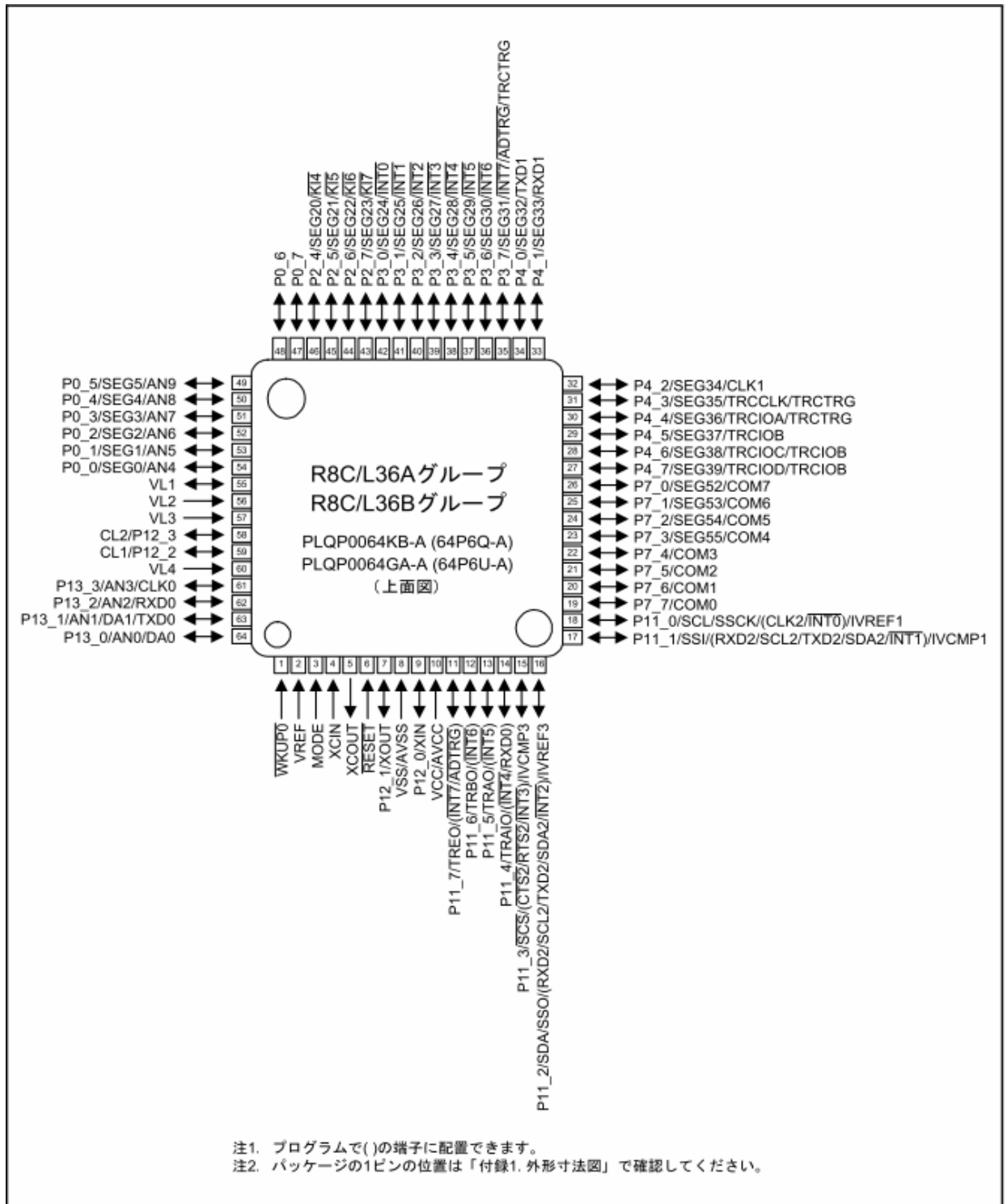
図3.2 R8C/L36Aグループピン配置図
