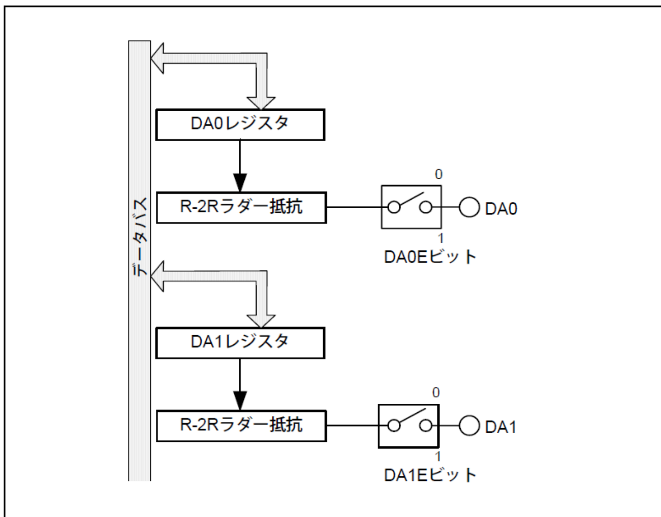
図4.3 R8C/L36AグループのD/Aコンバータブロック図
