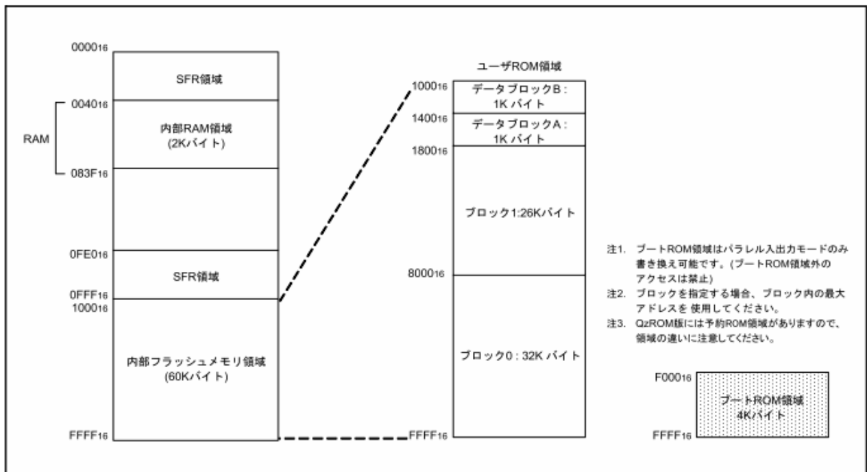
図3.4 38D2グループのフラッシュメモリ配置図
