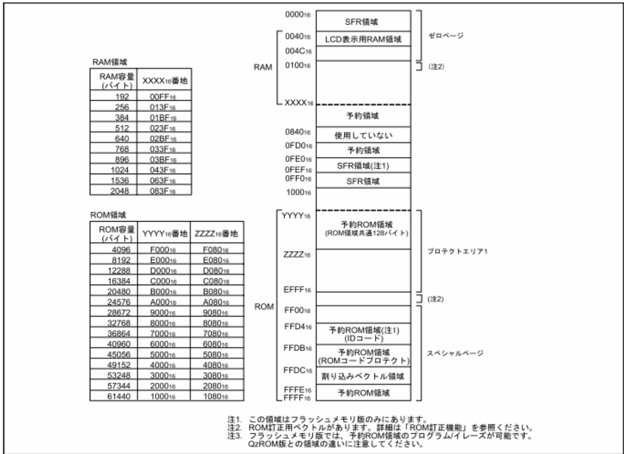
図3.3 38D2グループのメモリ配置図
