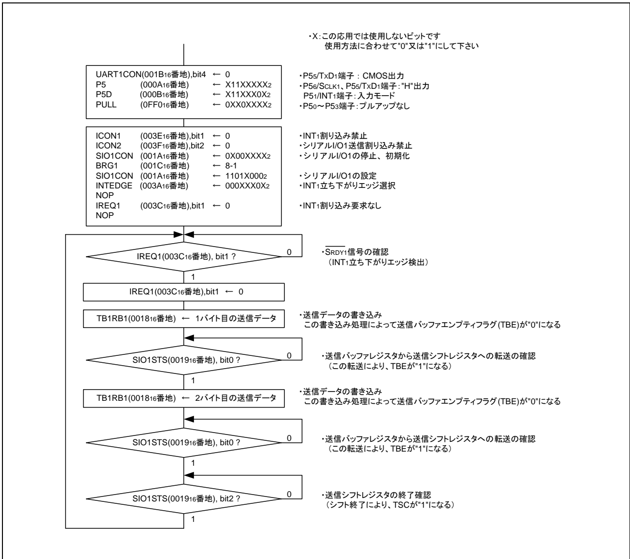
図 3.5 送信側の制御手順
