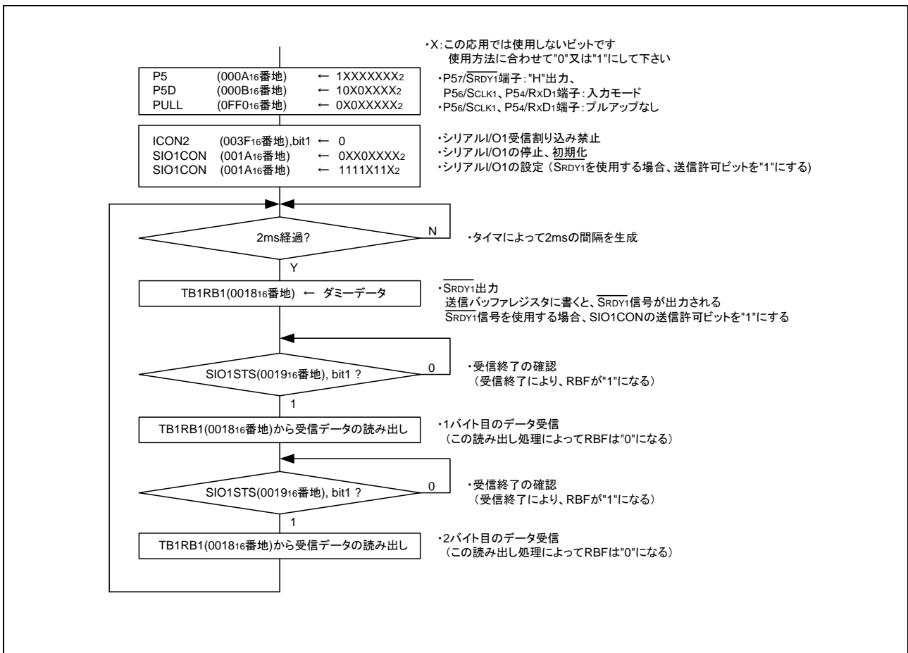
図 3.6 受信側の制御手順
