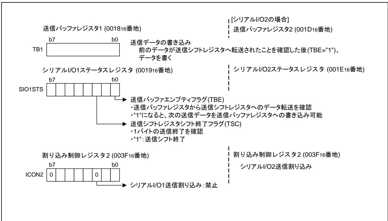
図 3.3 送信側関連レジスタの設定
