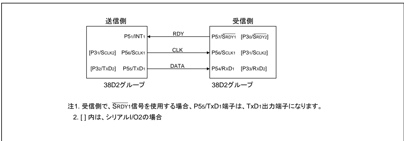
図 3.1 接続図
