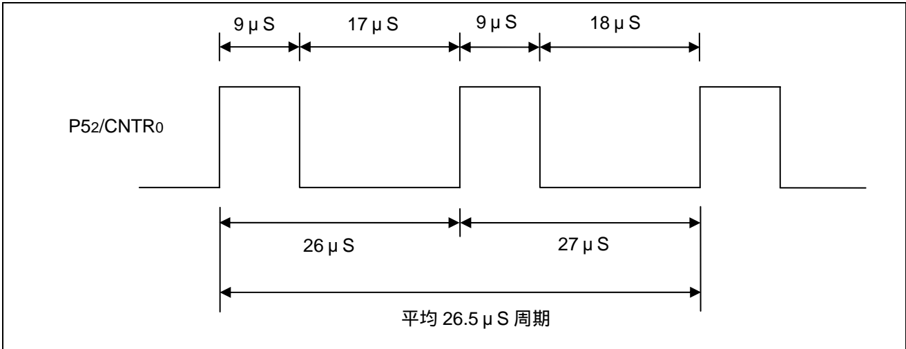
図 2. 周期 26.5 \mu S の搬送波
