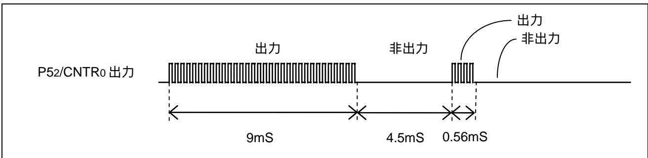
図 3. P52/CNTR0 出力波形
