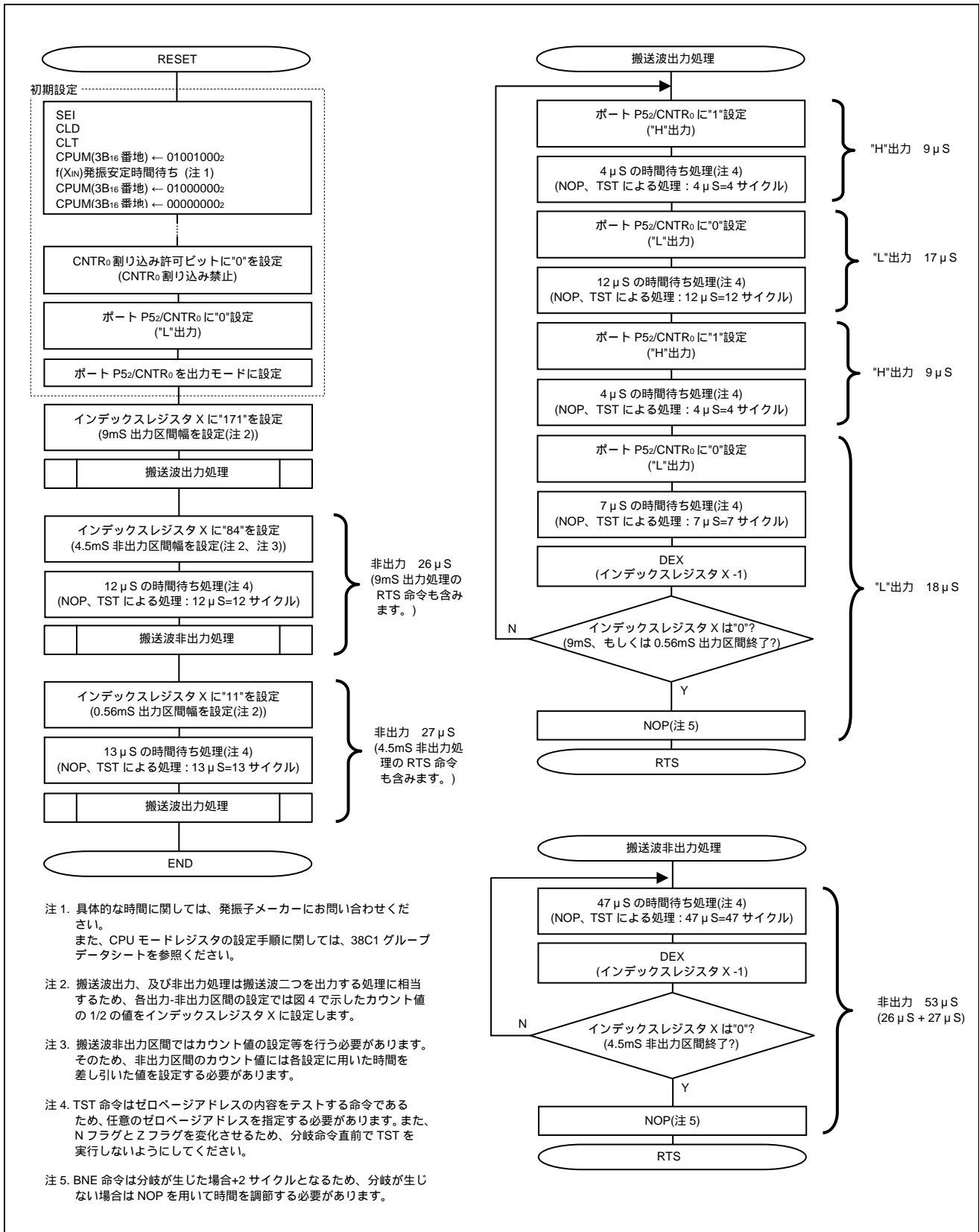
図 6. 制御手順例
