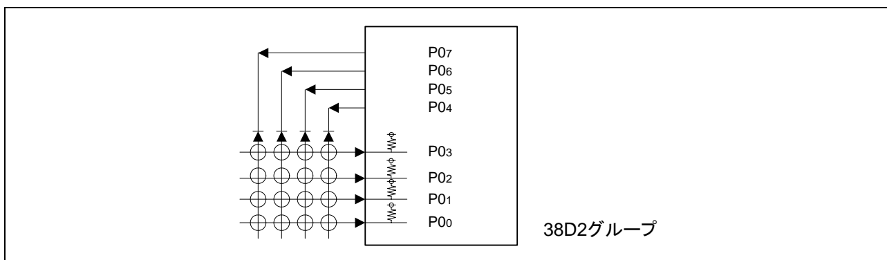
図 3.1 接続図
