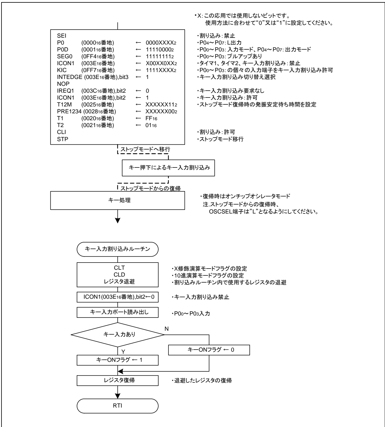
図 3.4 制御手順
