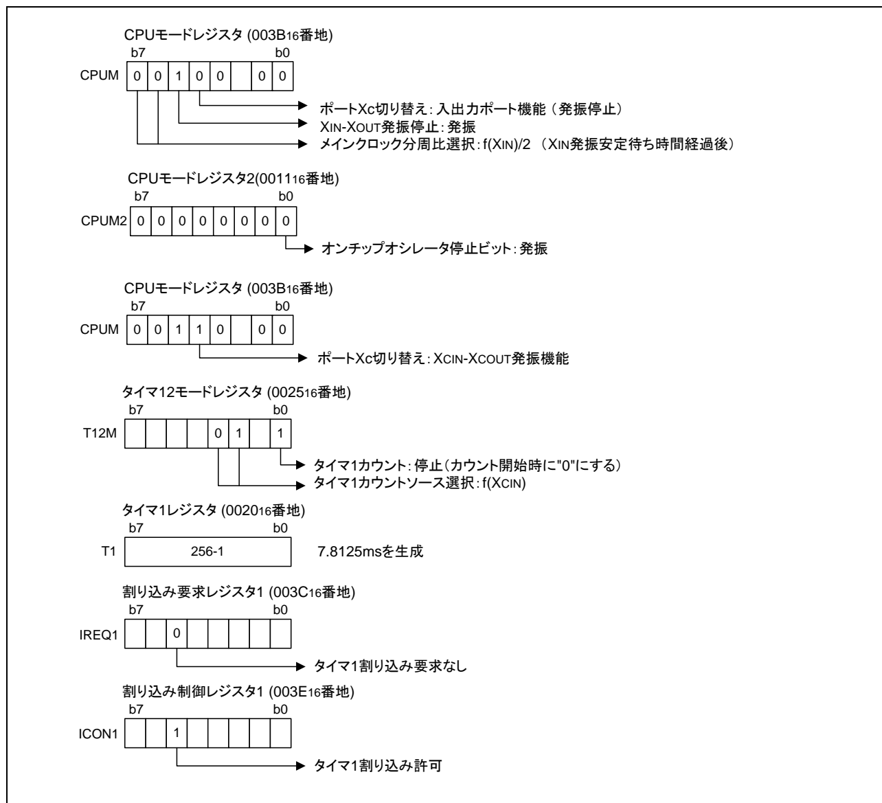
図 3.2 関連レジスタの設定
