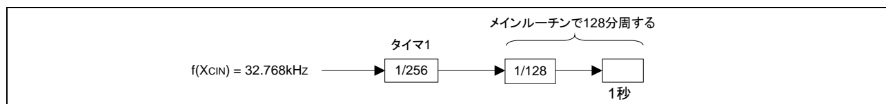
図 3.1 タイマの接続と分周比
