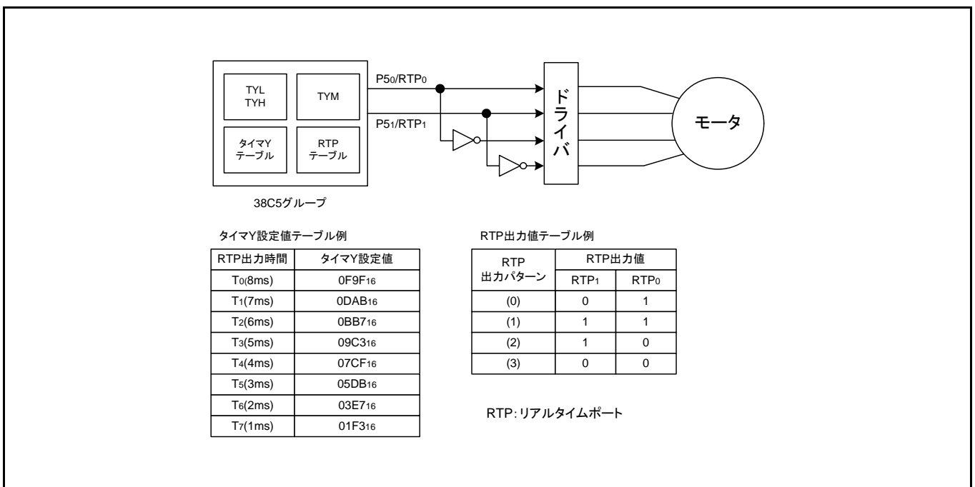
図 3.1 接続図、タイマ Y 設定値テーブル例及び RTP 出力値テーブル例
