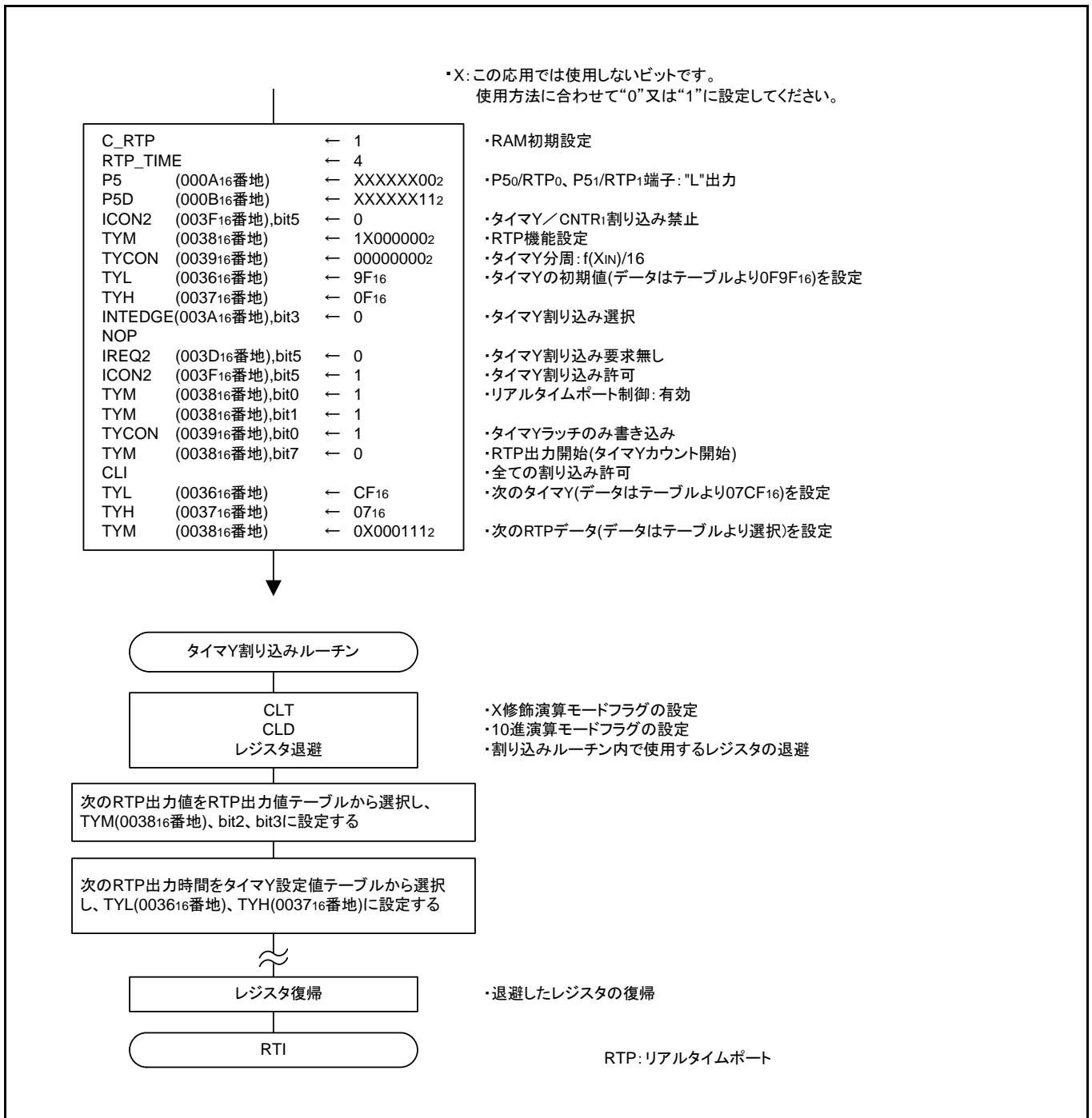
図 3.4 制御手順
