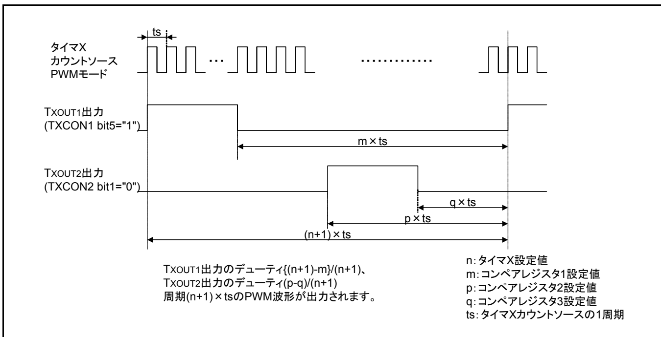
図 3.2 PWM(TxOUT1/TxOUT2)波形図
