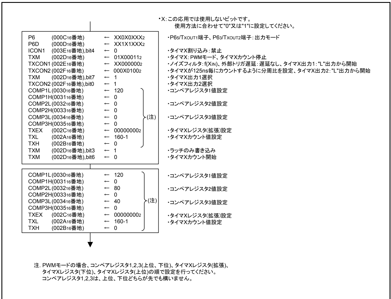
図 3.5 制御手順
