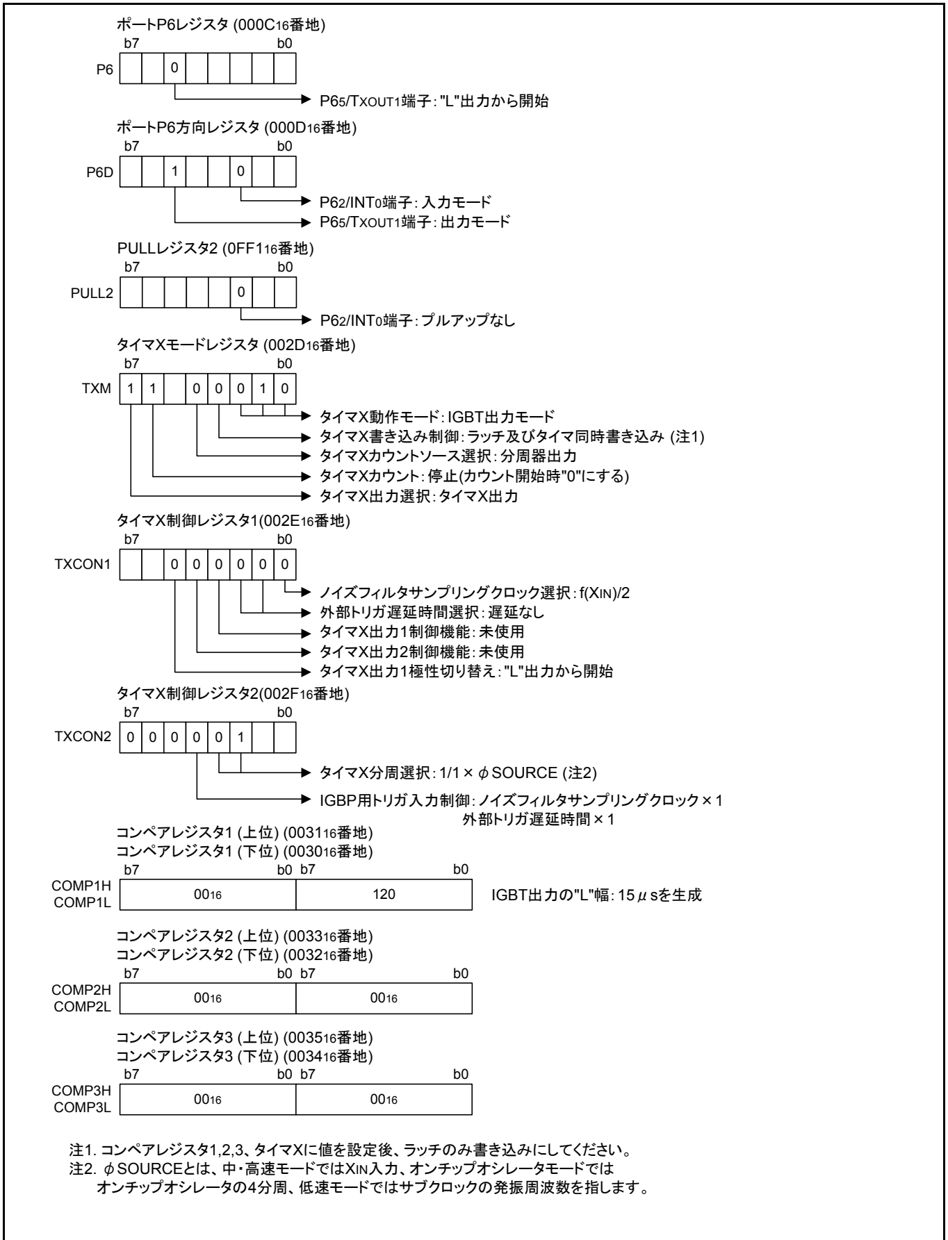
図 3.3 関連レジスタの設定(1)
