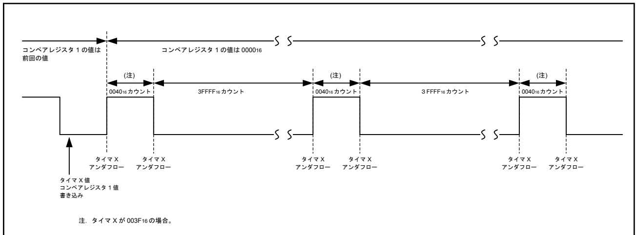
図 4.1 コンペアレジスタ 1 に 0000 16 を設定した場合 (前回の値は 0000 16 以外) の IGBT 制御信号出力例
