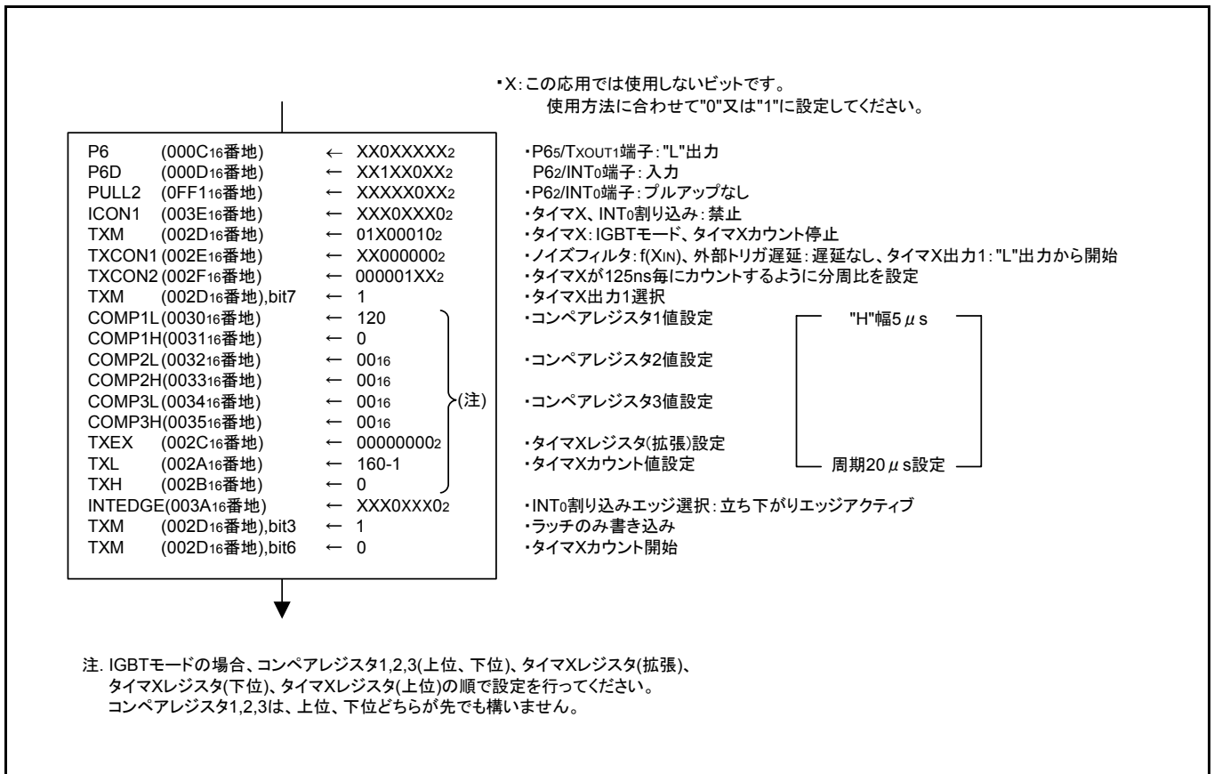
図 3.5 制御手順
