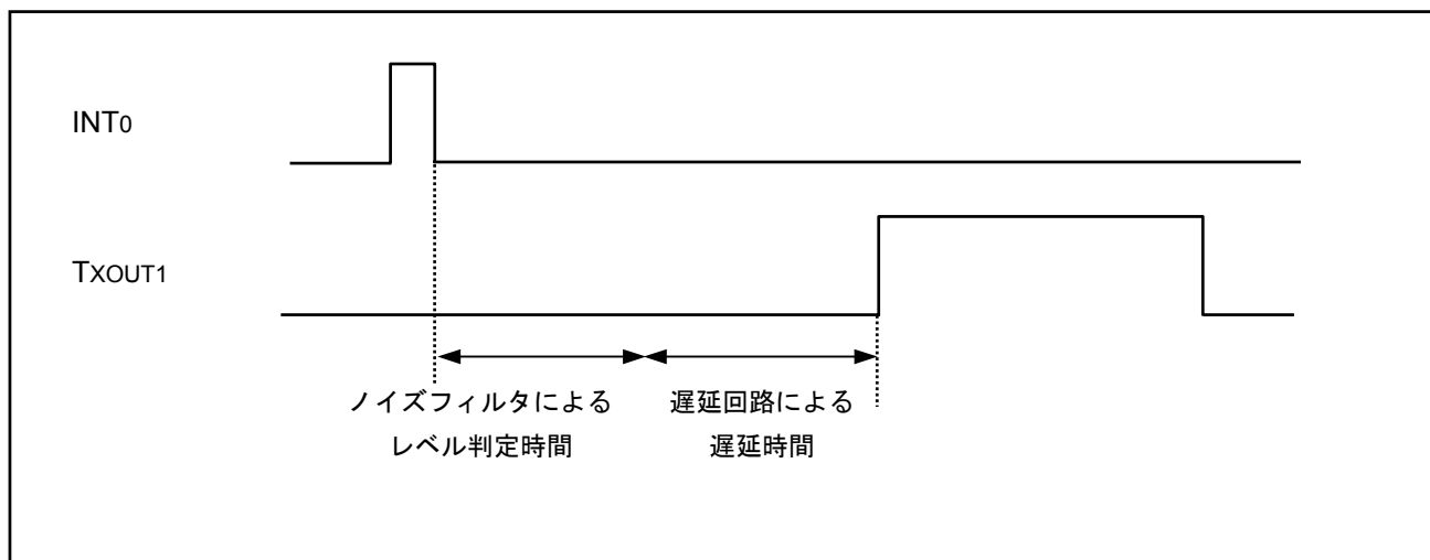
図 4.3 INT0 端子へのトリガ入力による TxOUT1 端子からの IGBT 制御信号出力例
