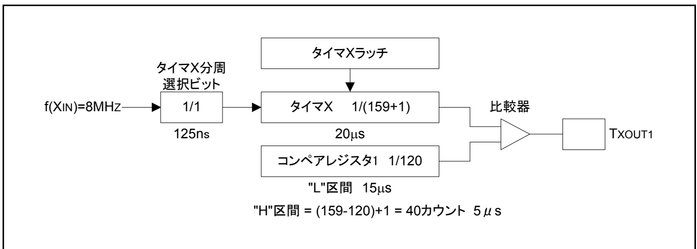
図 3.1 タイマの接続と分周比の設定
