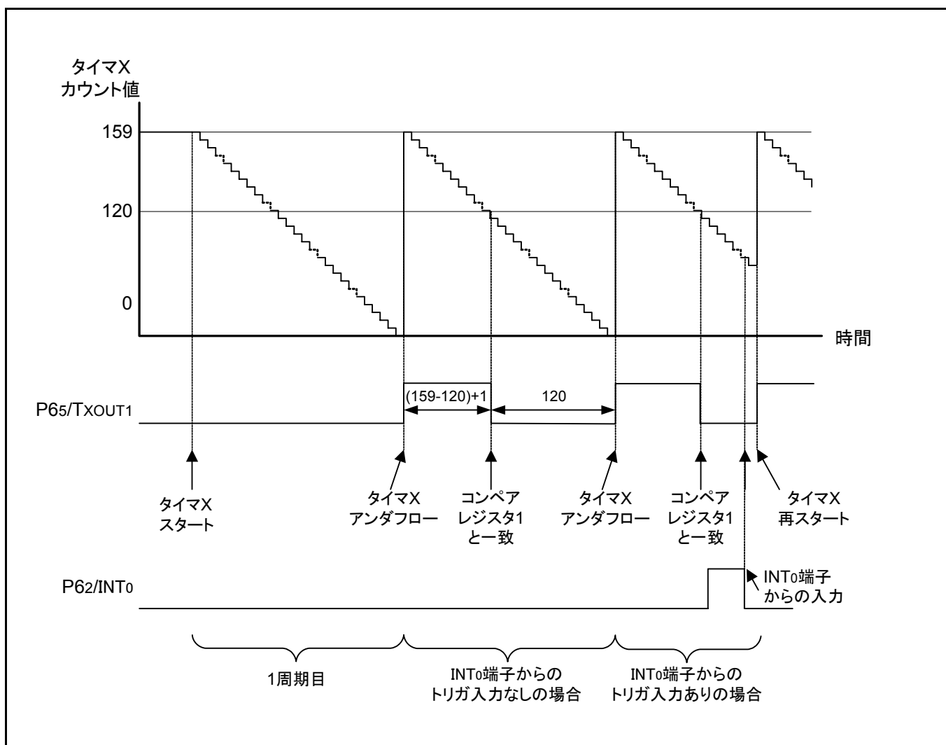
図 3.2 TXOUT1 出力波形
