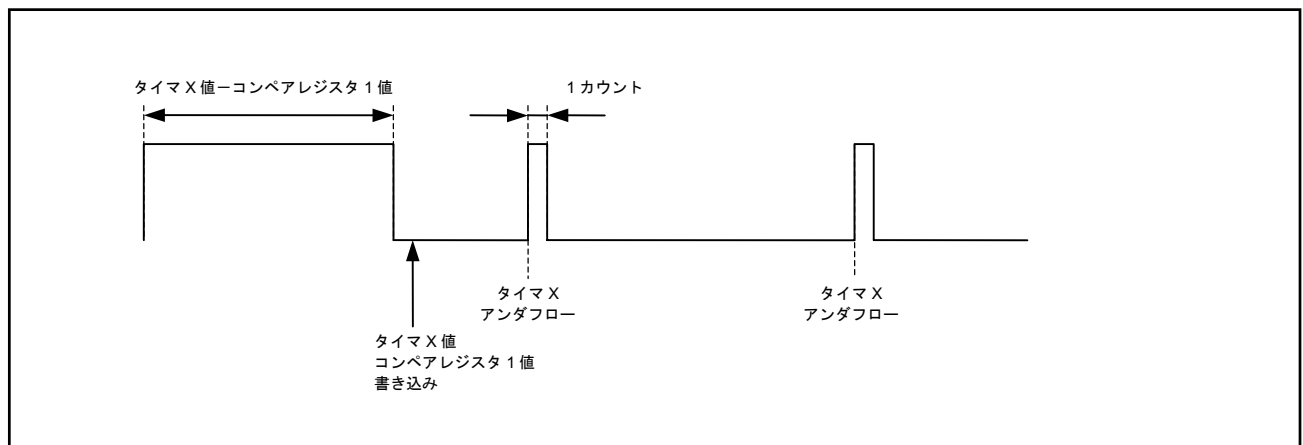
図 4.2 タイマ X 値とコンペアレジスタ 1 値を同じ値に設定した場合の IGBT 制御信号出力例
