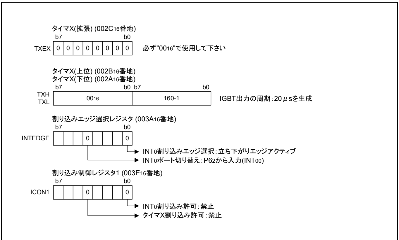
図 3.4 関連レジスタの設定(2)
