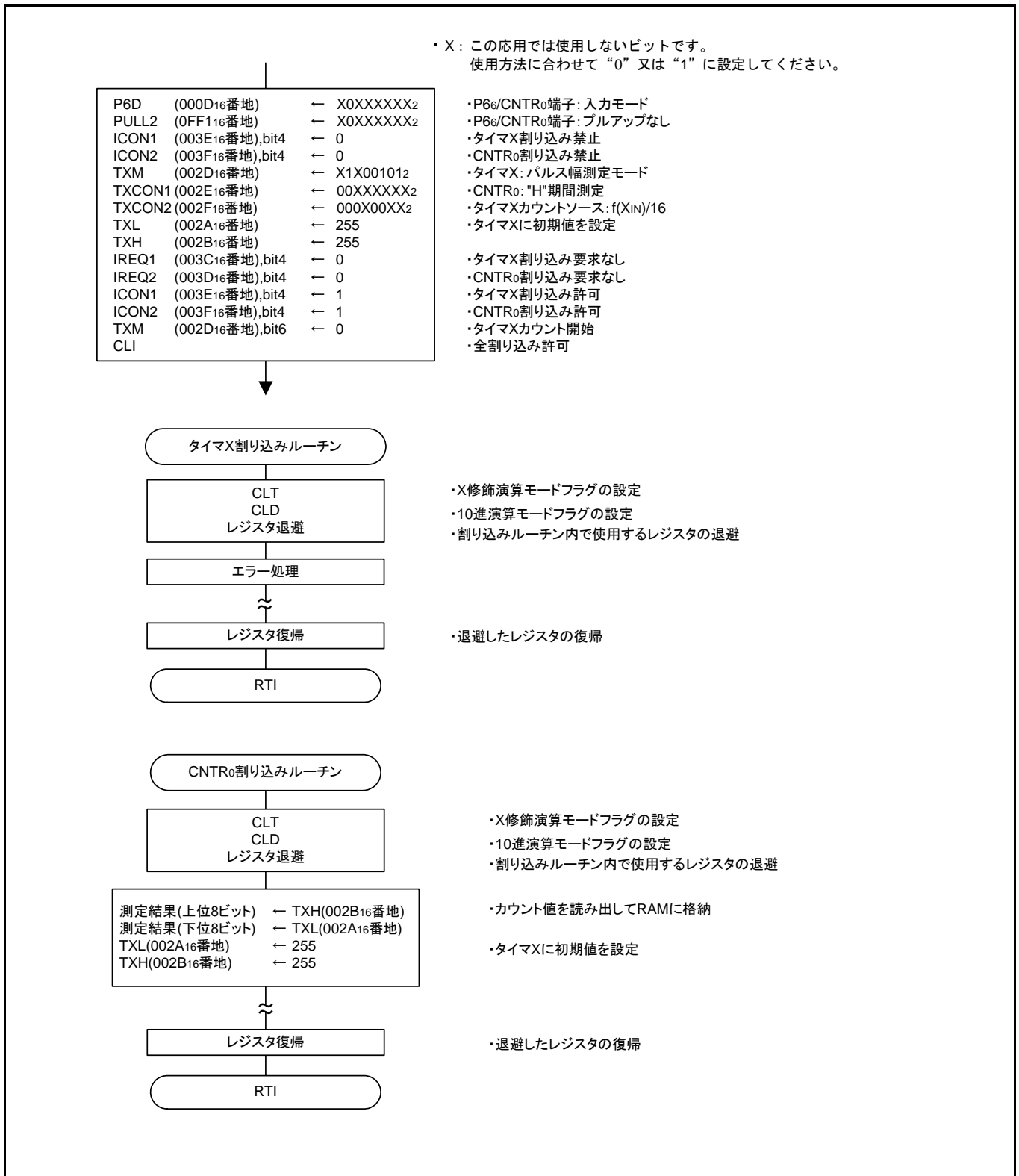
図 3.3 制御手順
