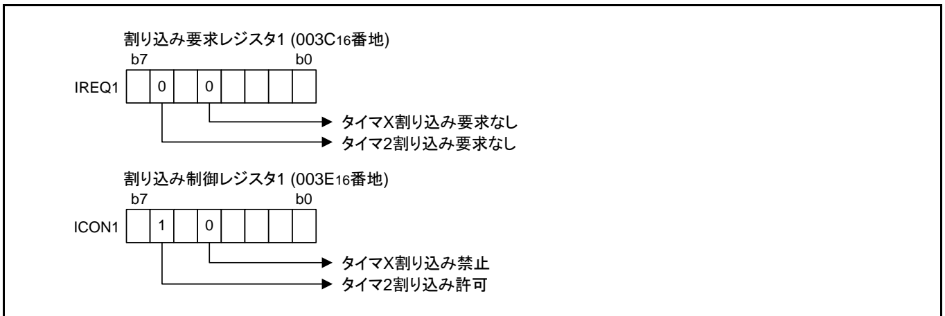
図 3.3 関連レジスタの設定(2)
