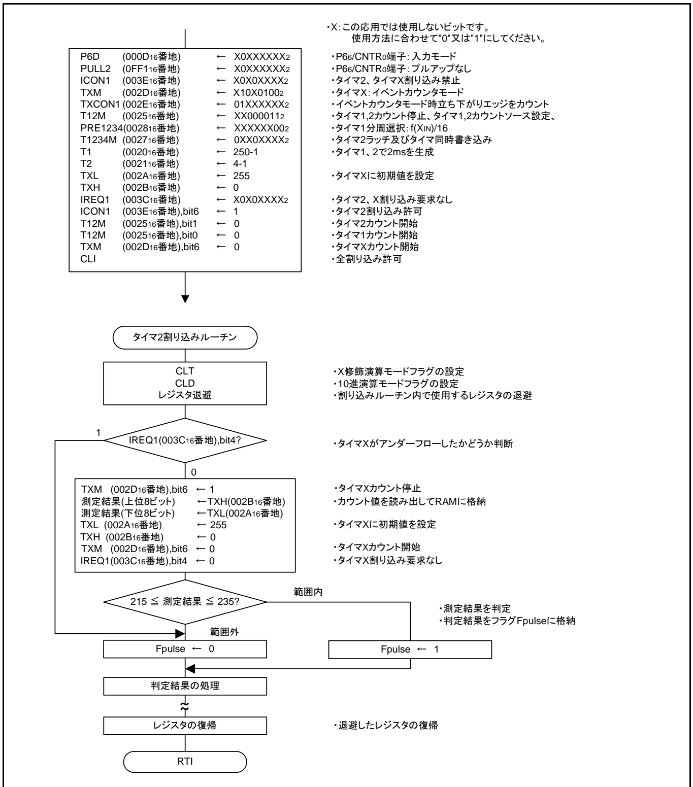
図 3.4 制御手順
