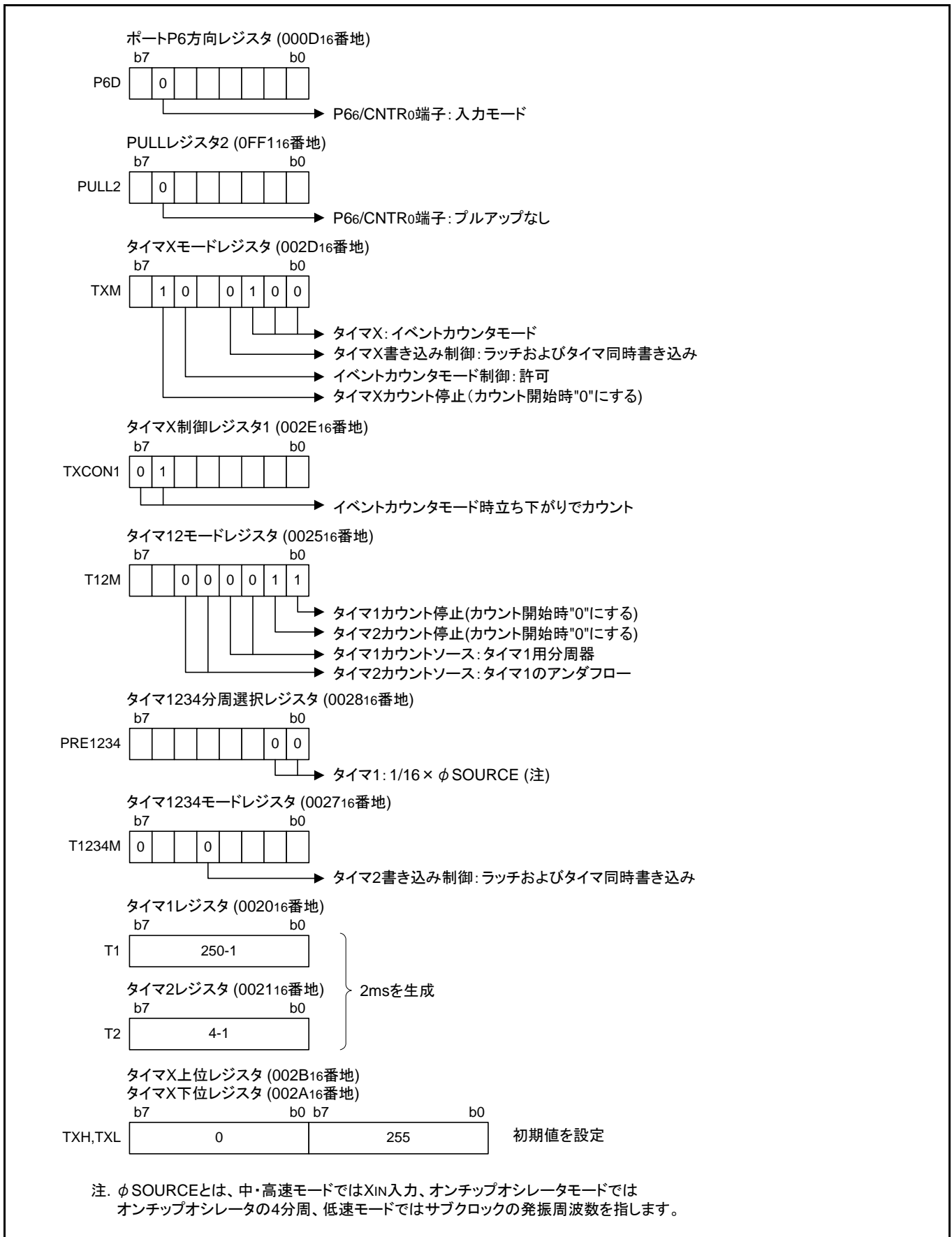
図 3.2 関連レジスタの設定(1)
