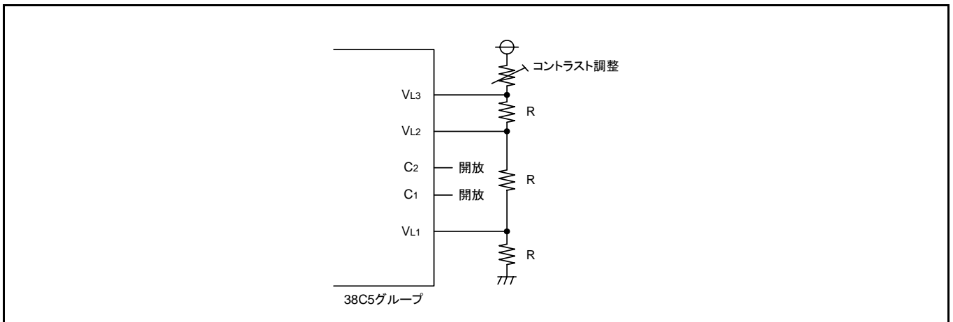
図 3.2 回路例(外付け分割抵抗使用時)
