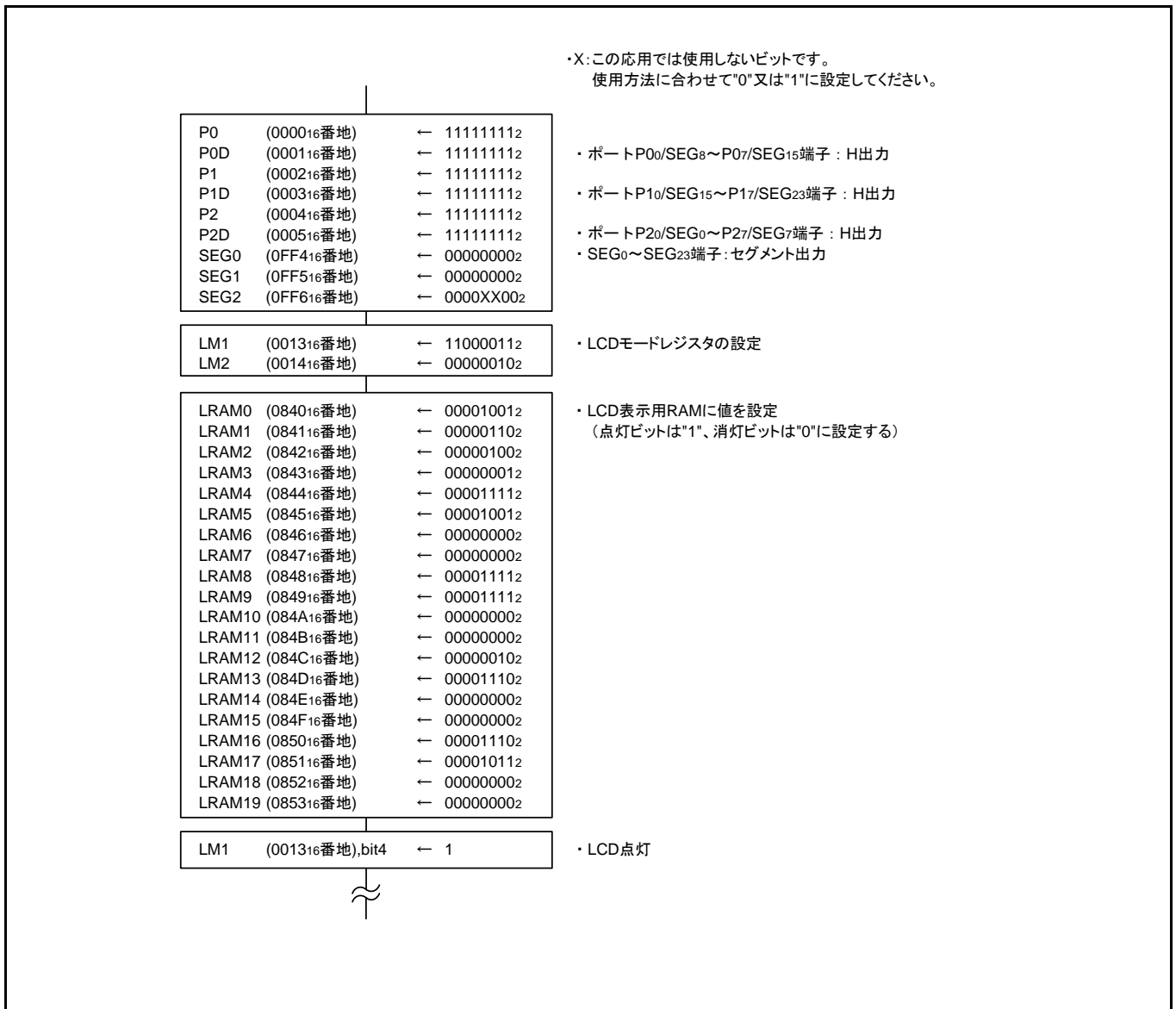
図 3.7 制御手順
