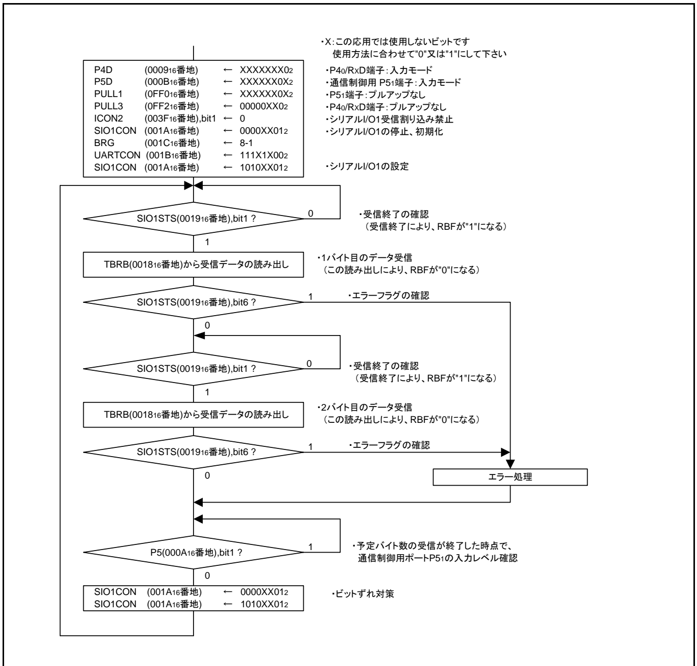
図 3.8 受信側の制御手順
