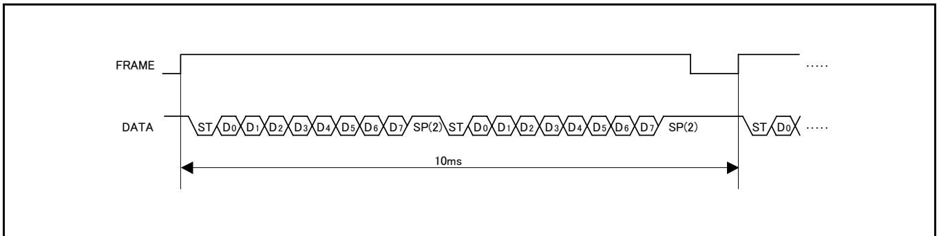
図 3.2 タイミング図
