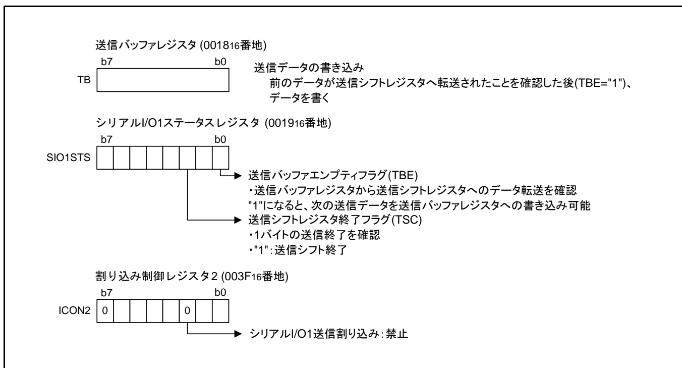
図 3.4 送信側関連レジスタの設定(2)
