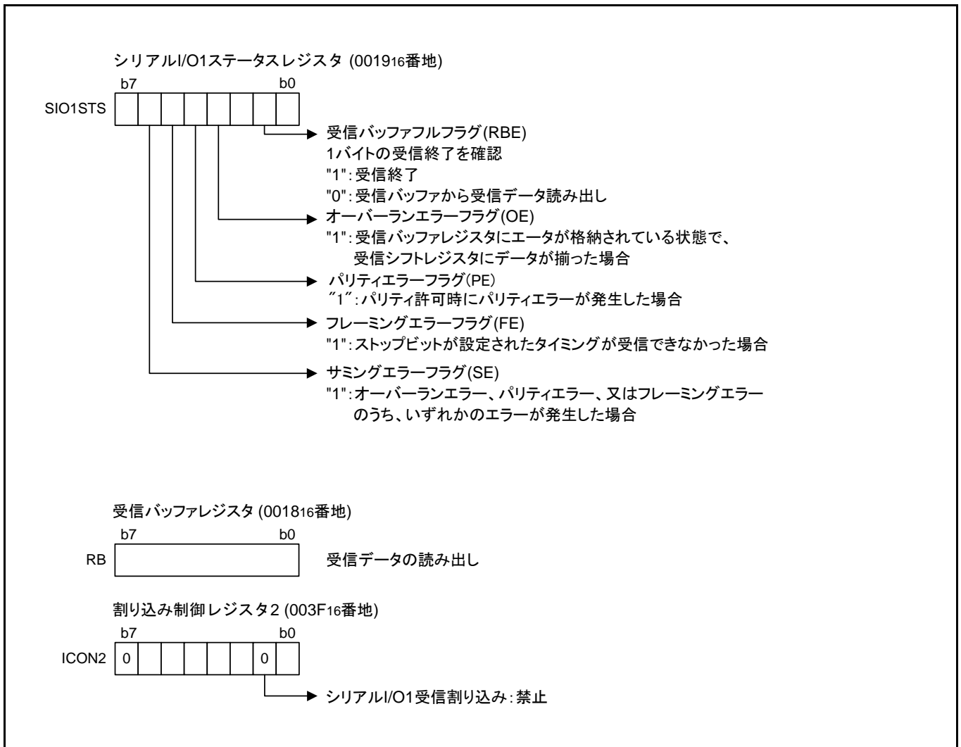
図 3.6 受信側関連レジスタの設定(2)
