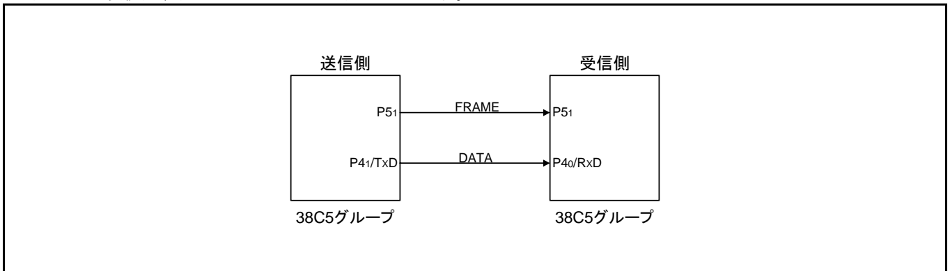
図 3.1 接続図
