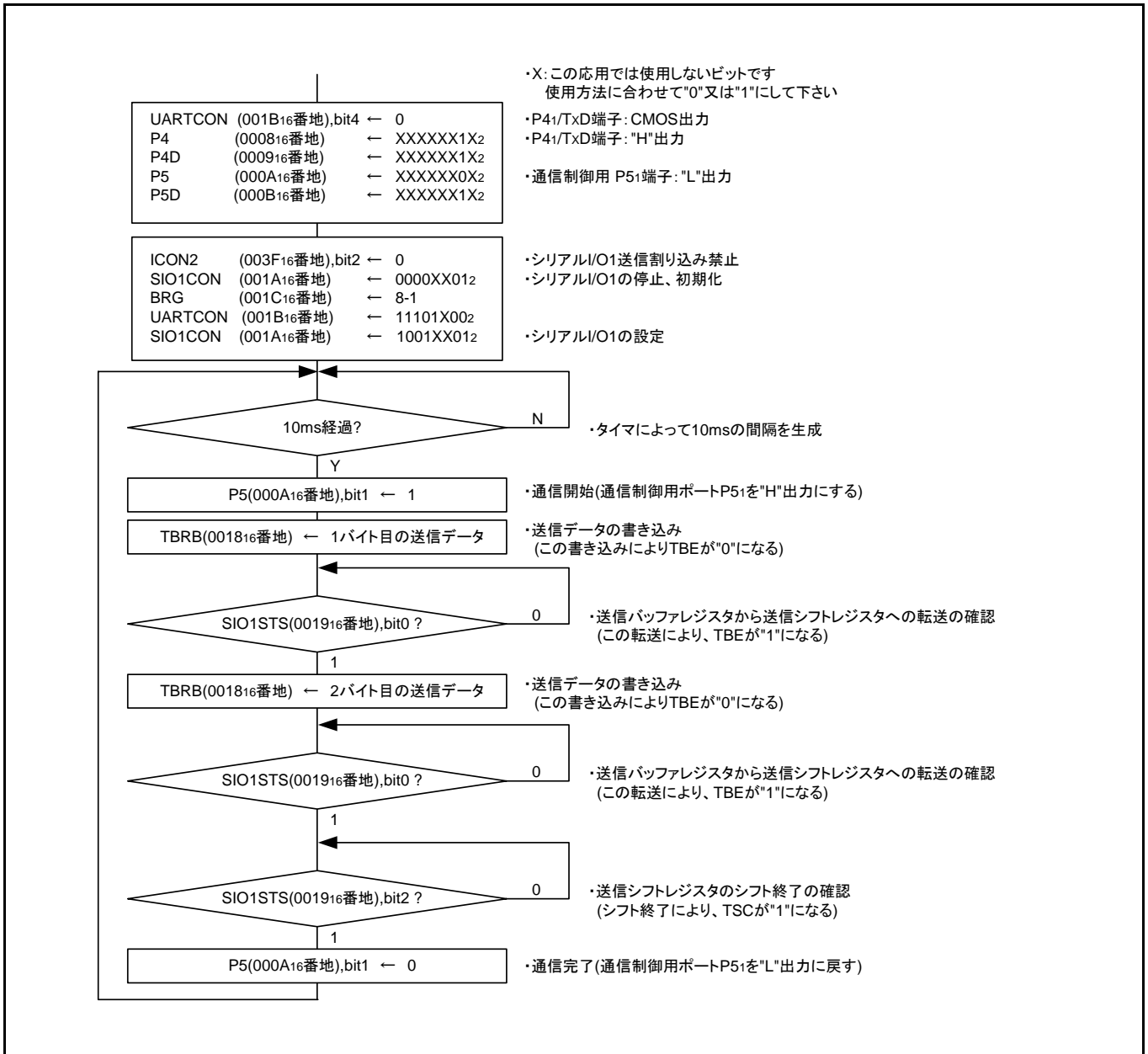
図 3.7 送信側の制御手順
