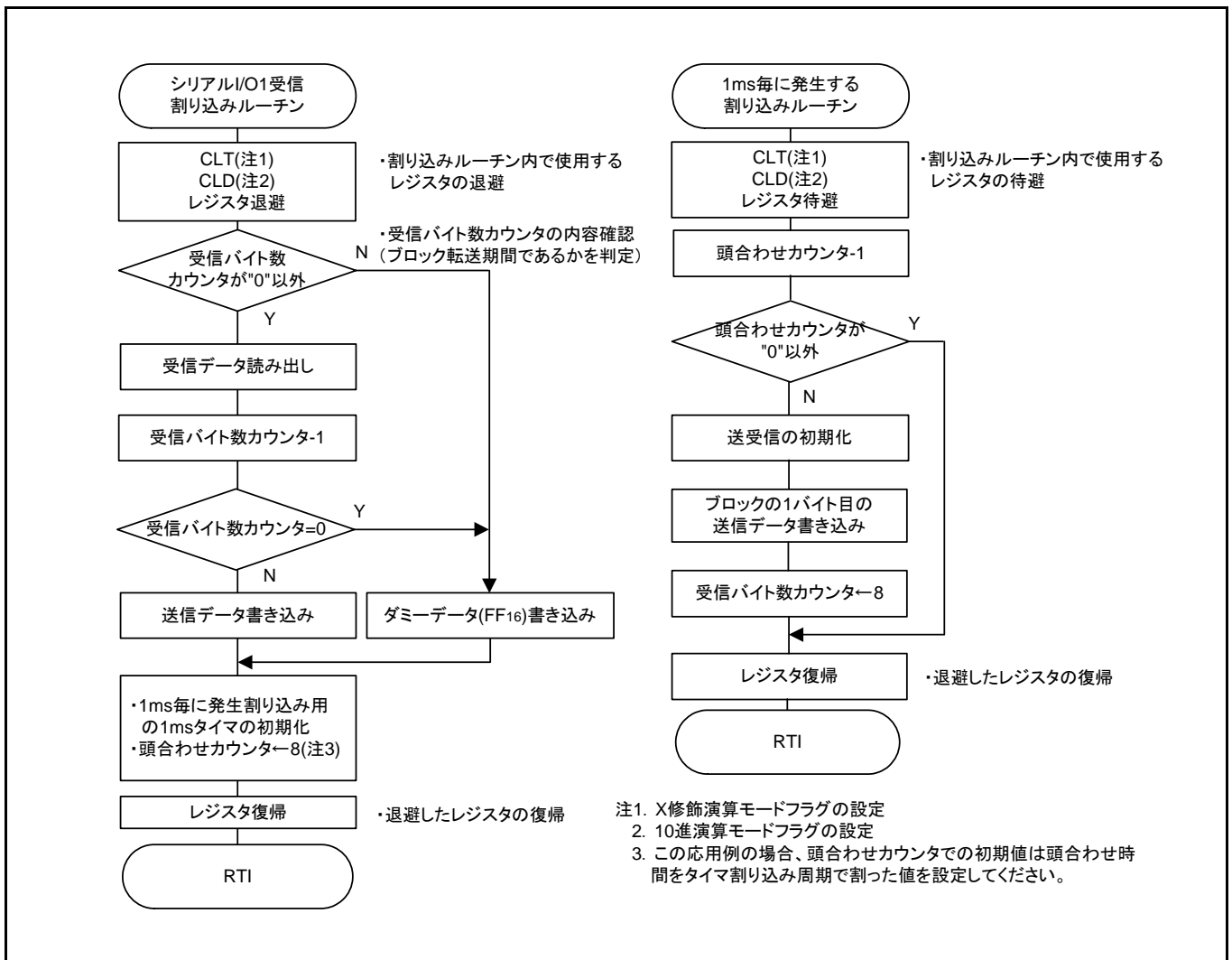
図 3.5 スレーブ側の制御手順
