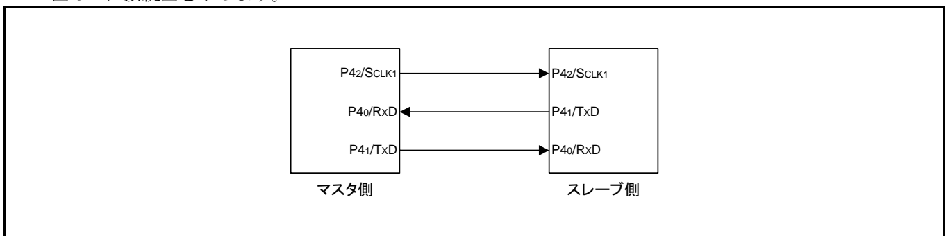
図 3.1 接続図
