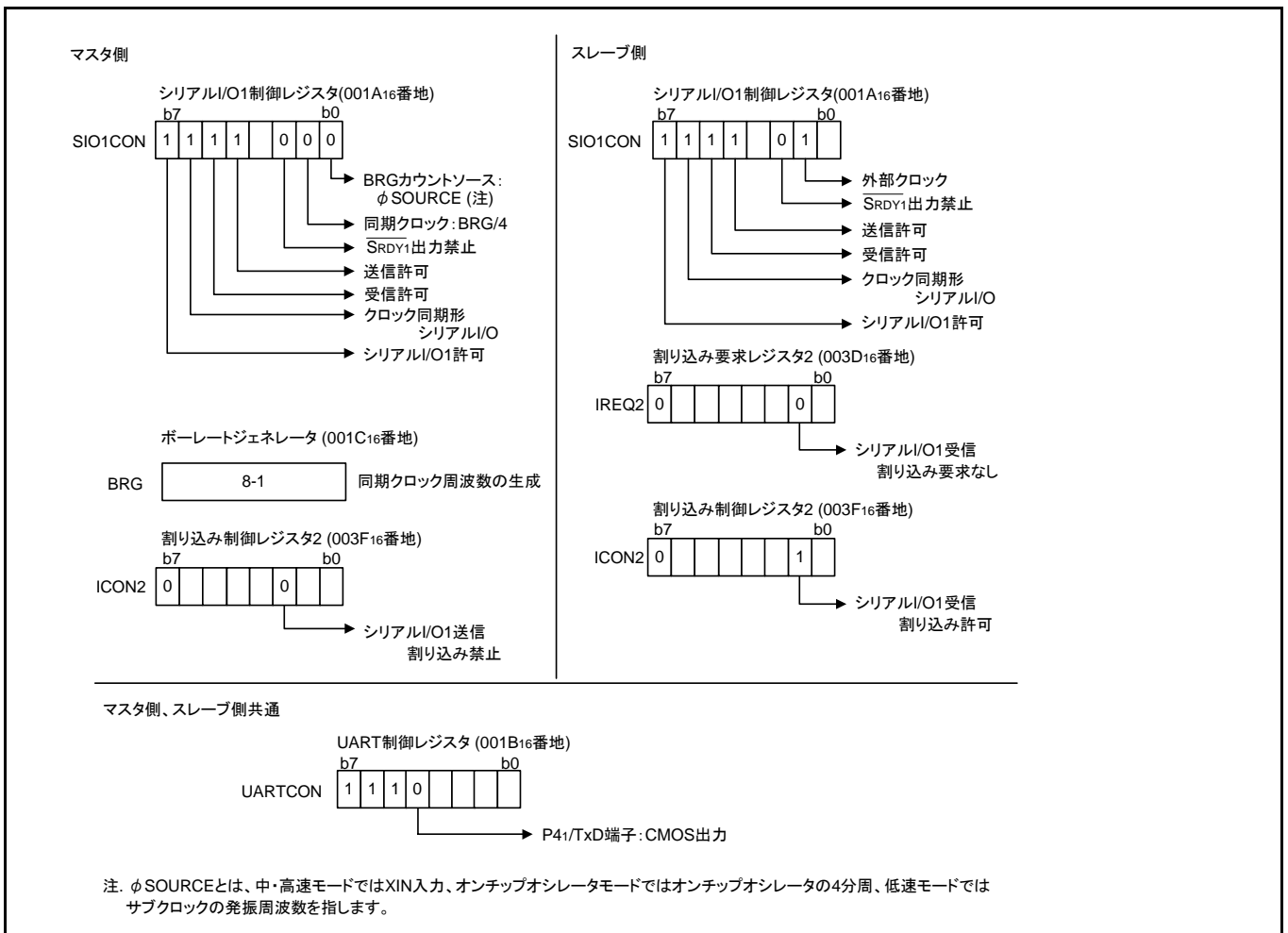
図 3.3 関連レジスタの設定
