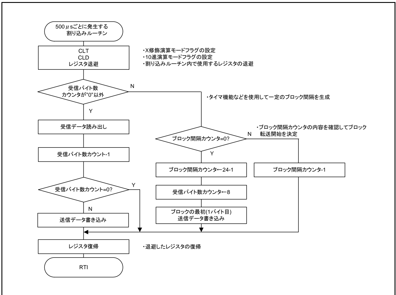
図 3.4 マスタ側の制御手順
