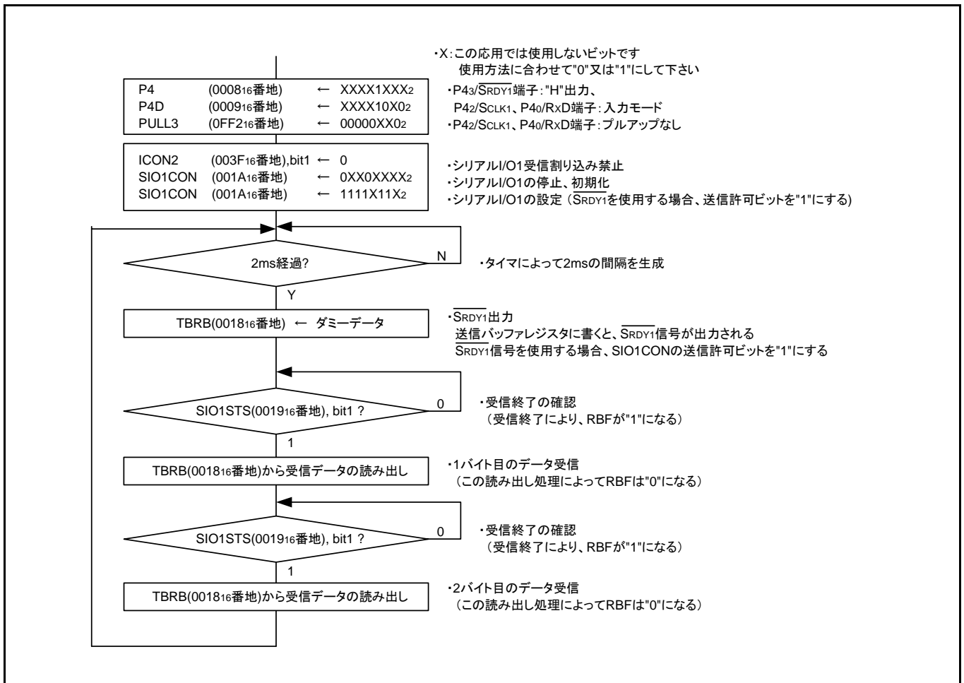
図 3.7 受信側の制御手順
