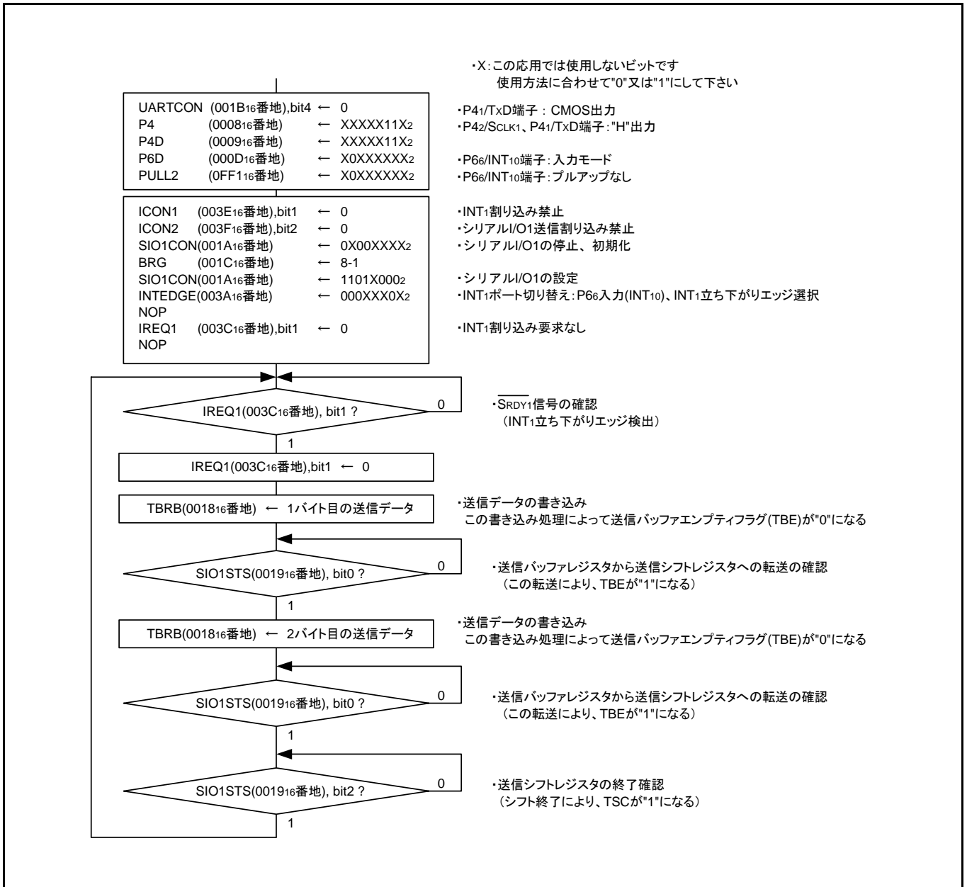
図 3.6 送信側の制御手順
