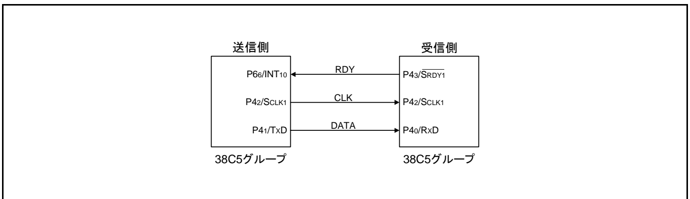
図 3.1 接続図
