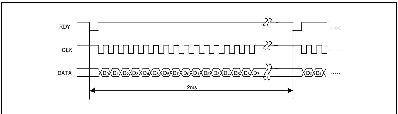
図 3.2 タイミング図
