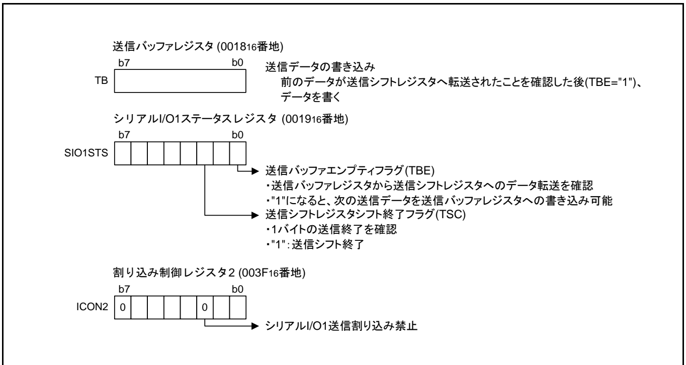
図 3.4 送信側関連レジスタの設定(2)
