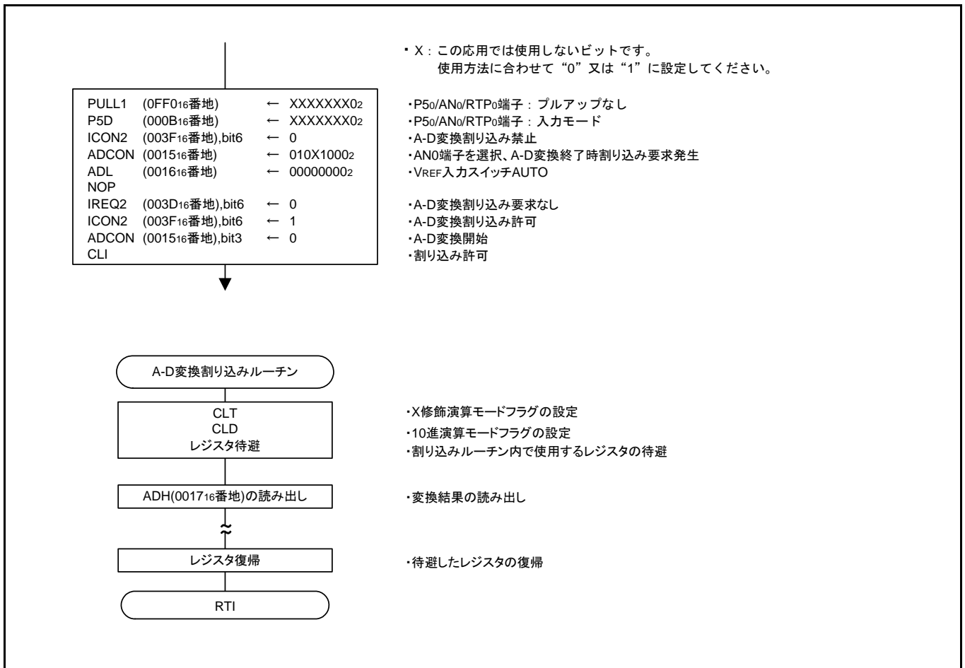
図 3.3 8 ビット A-D モード時の制御手順
