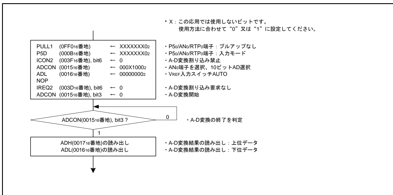
図 3.3 10 ビット A-D モード時の制御手順
