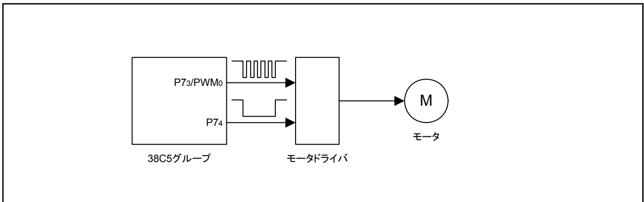
図 3.1 接続図
