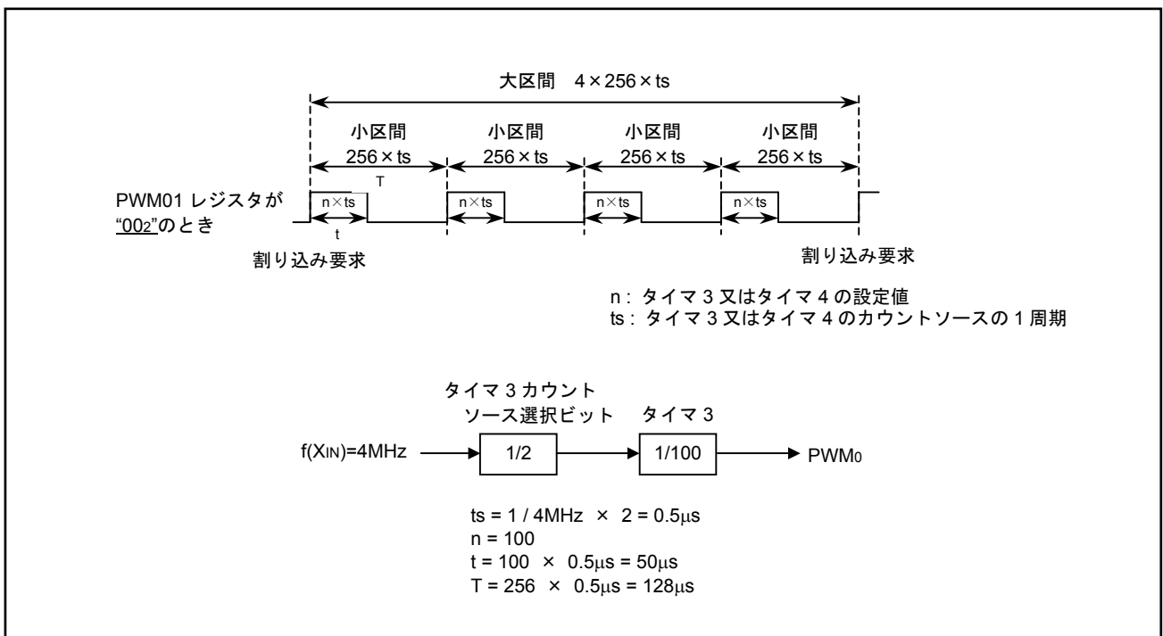
図 3.2 PWM0 および PWM1 の出力波形図
