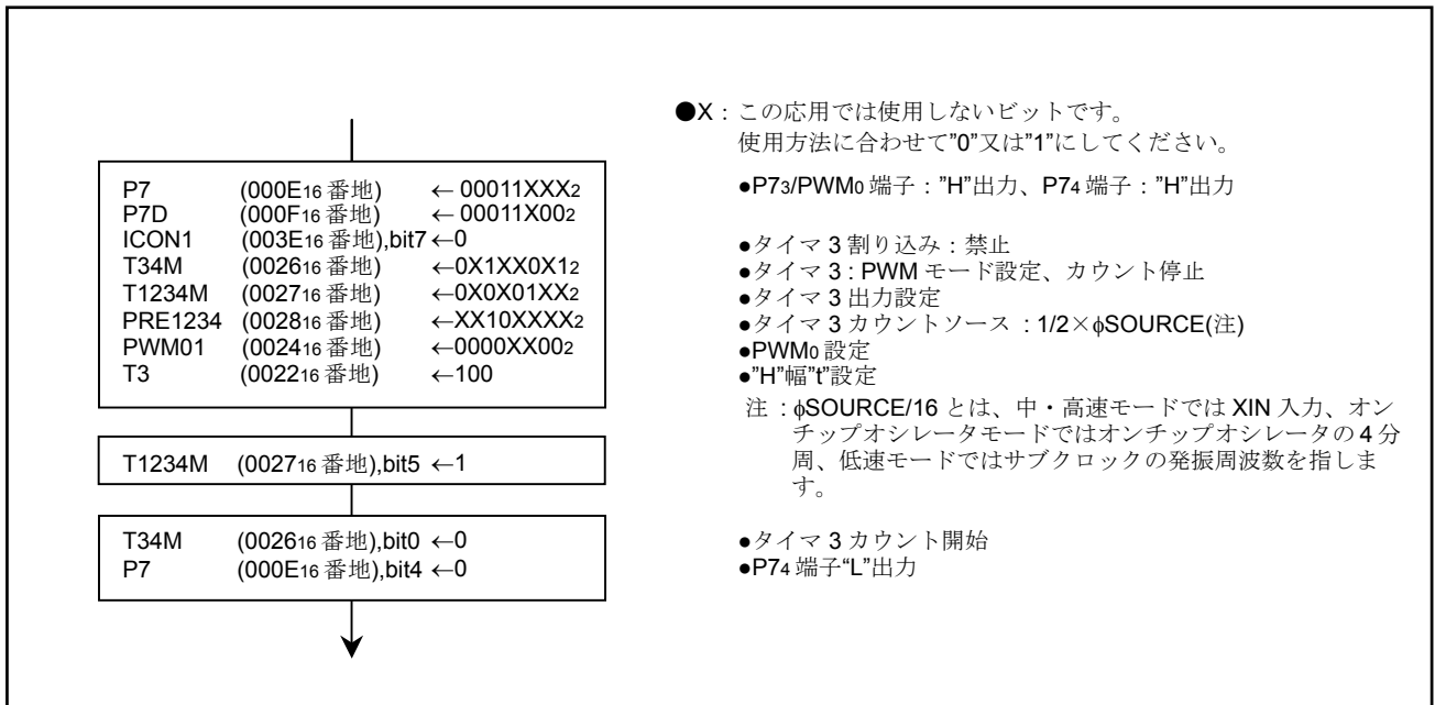
図 3.4 制御手順
