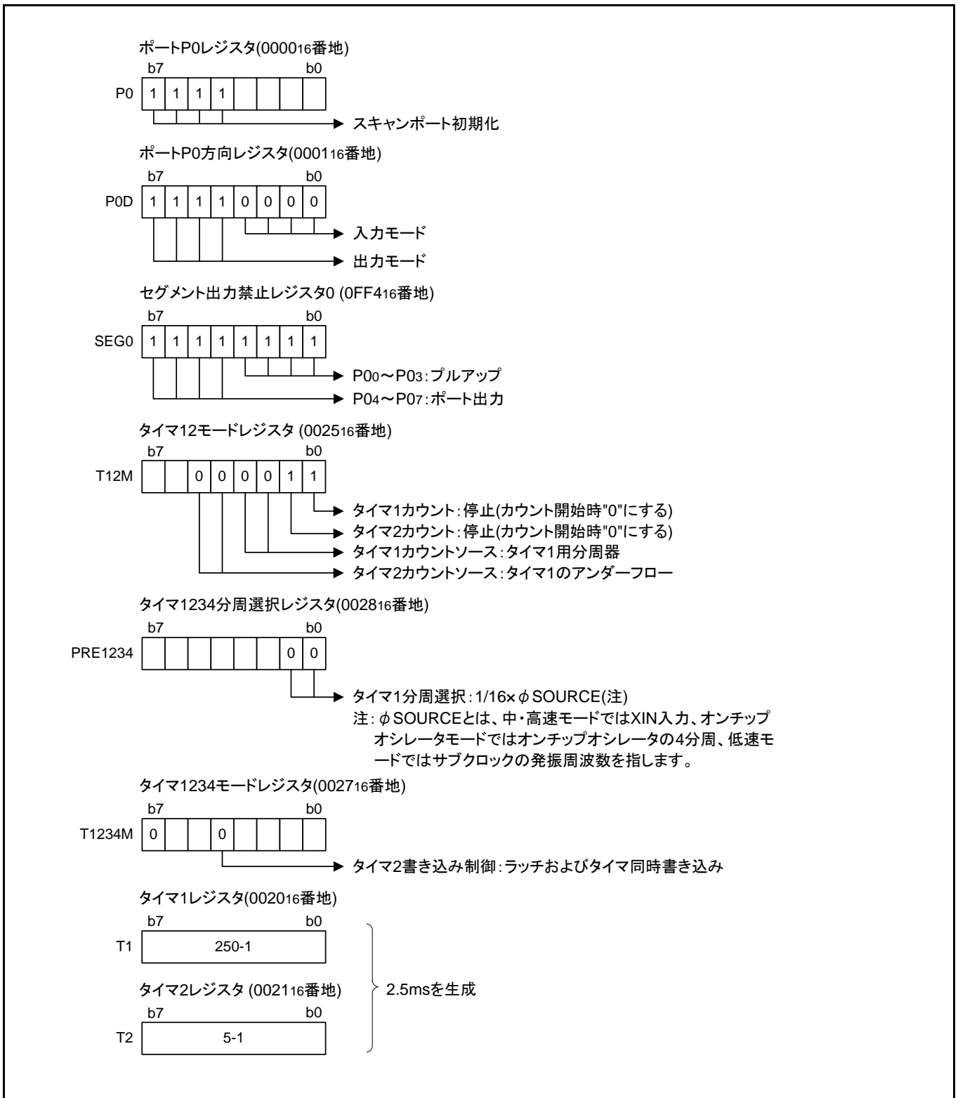
図 3.2 関連レジスタの設定 1
