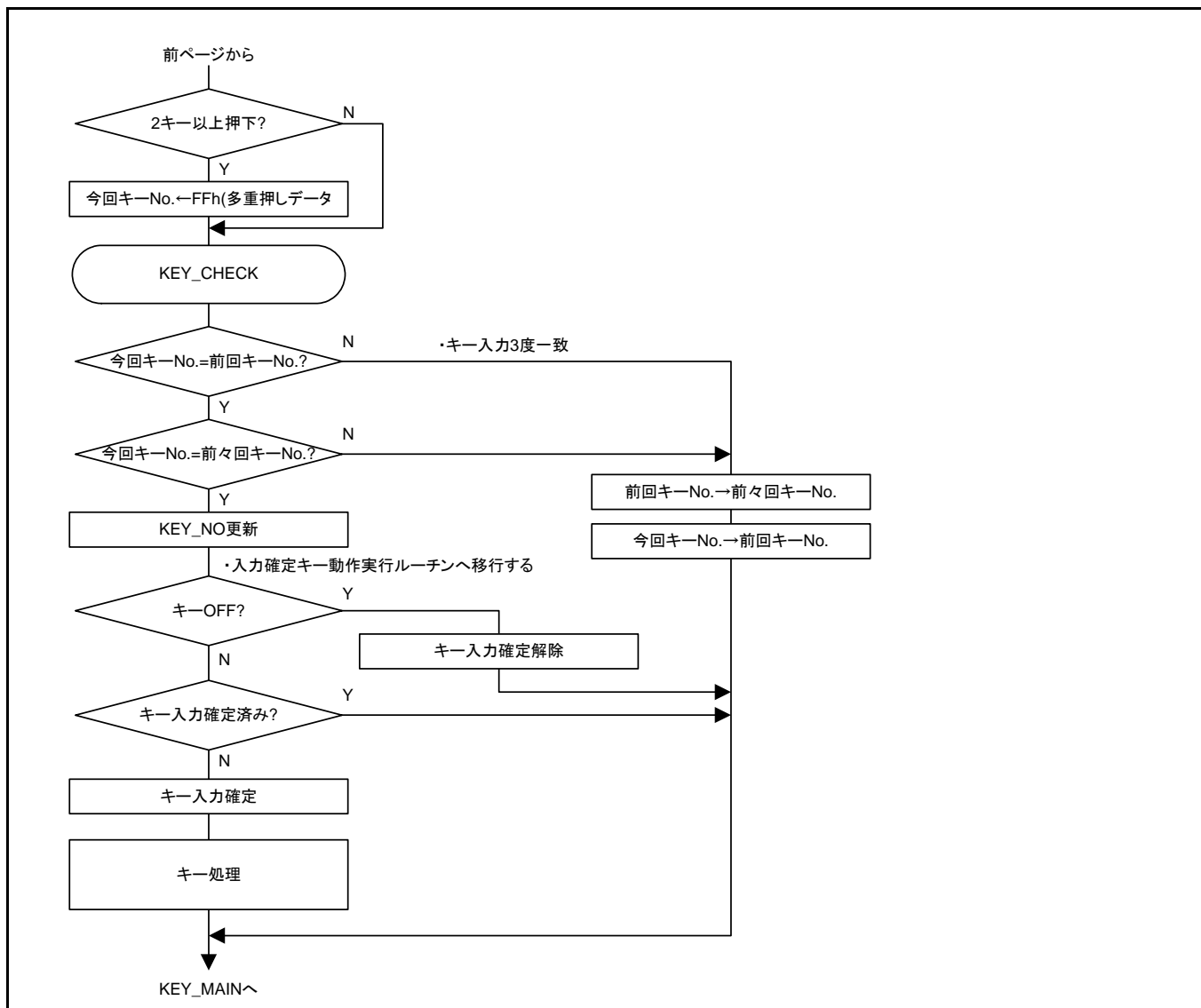
図 3.5 制御手順 2
