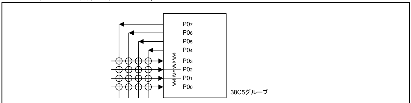
図 3.1 接続図
