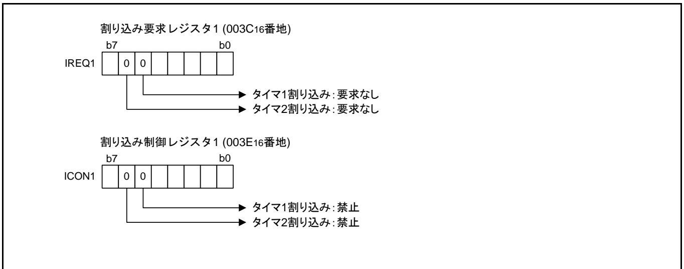
図 3.3 関連レジスタの設定 2
