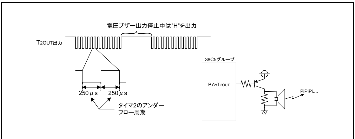
図 3.1 出力波形図及び周辺回路例
