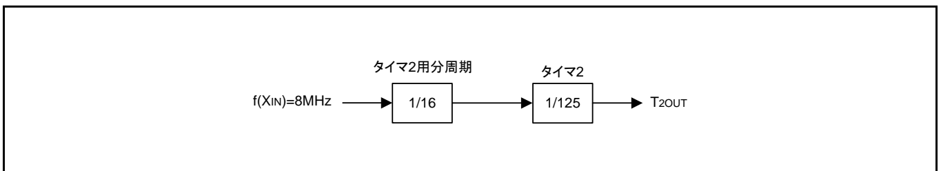
図 3.2 タイマの接続と分周比
