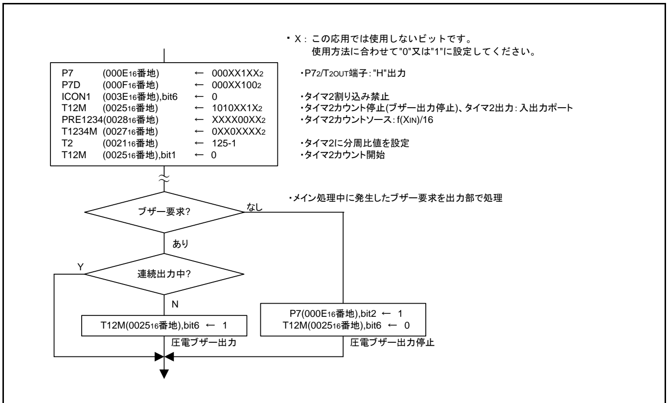
図 3.4 制御手順
