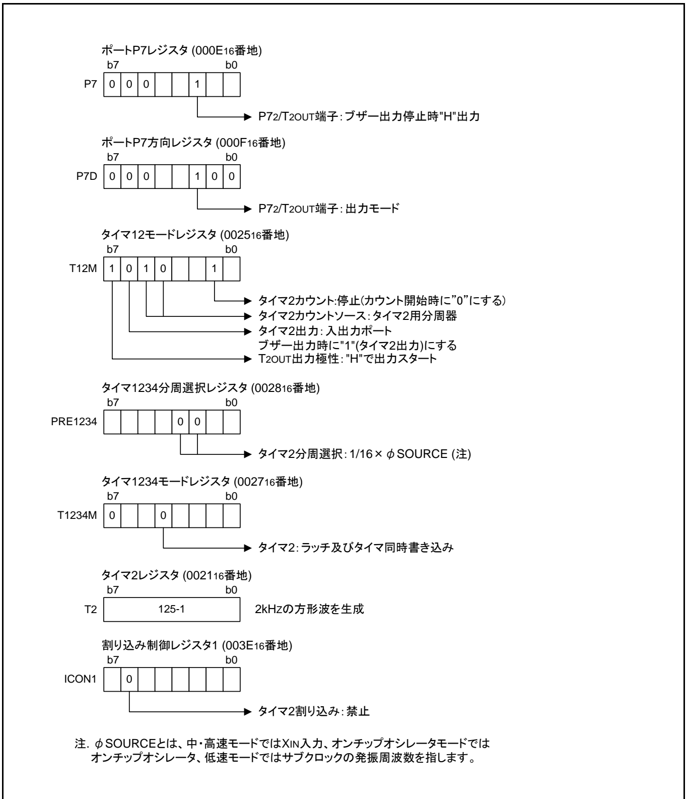
図 3.3 関連レジスタの設定
