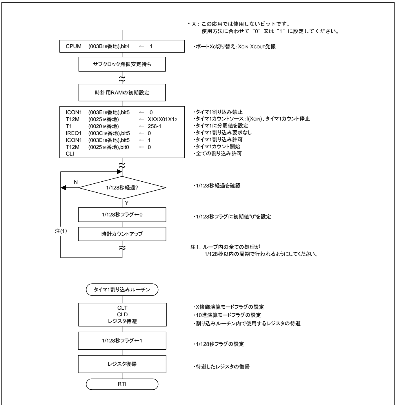
図 3.3 制御手順
