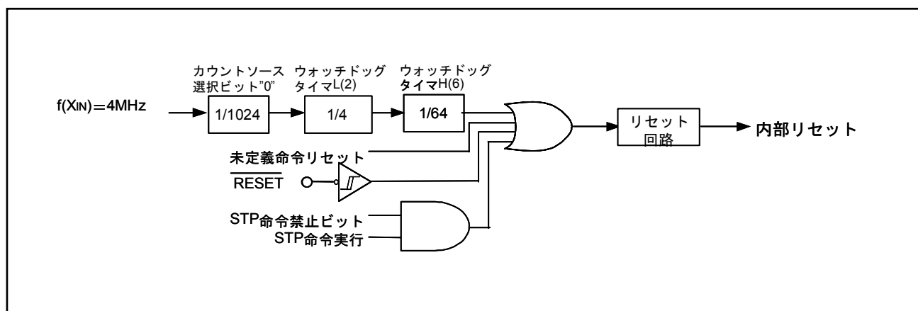
図 3.1 ウォッチドッグタイマの接続と分周比の設定
