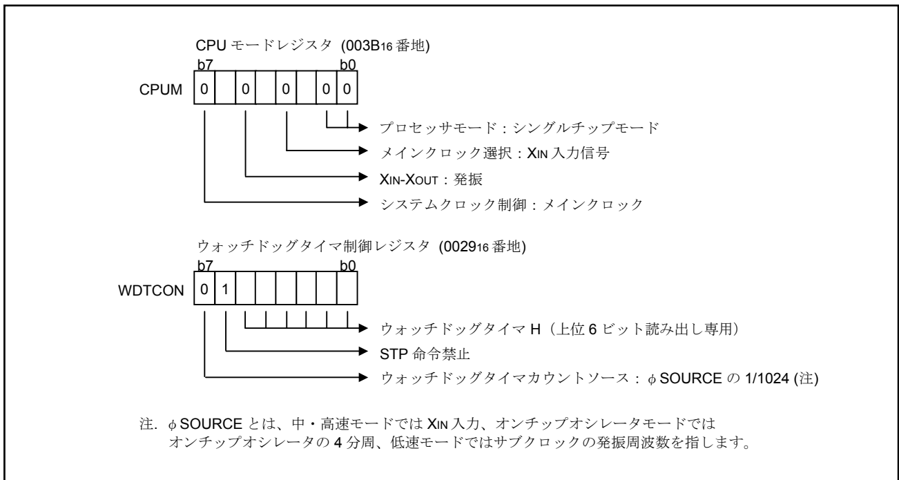
図 3.2 関連レジスタの設定
