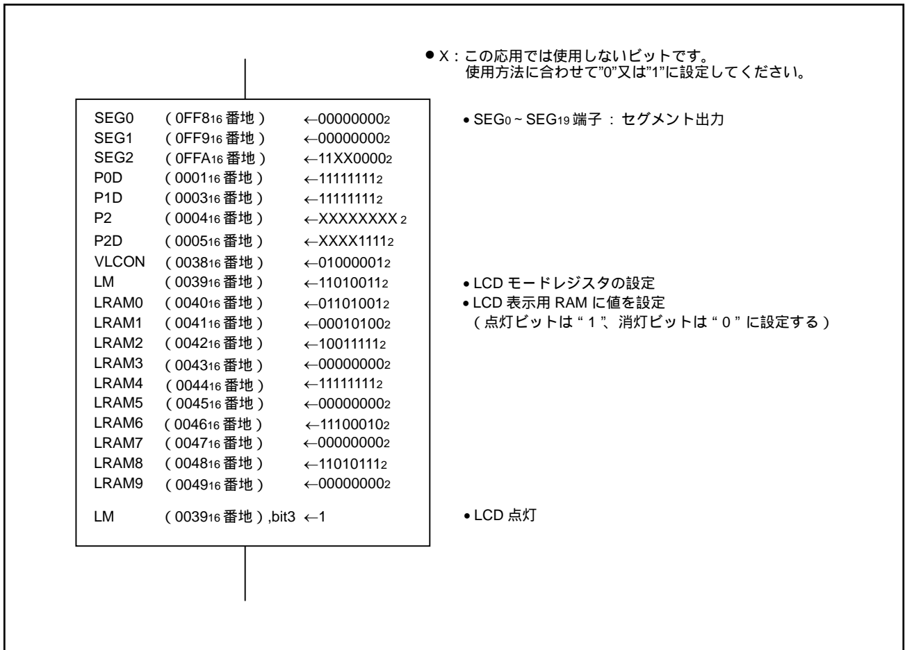
図 3.7 制御手順
