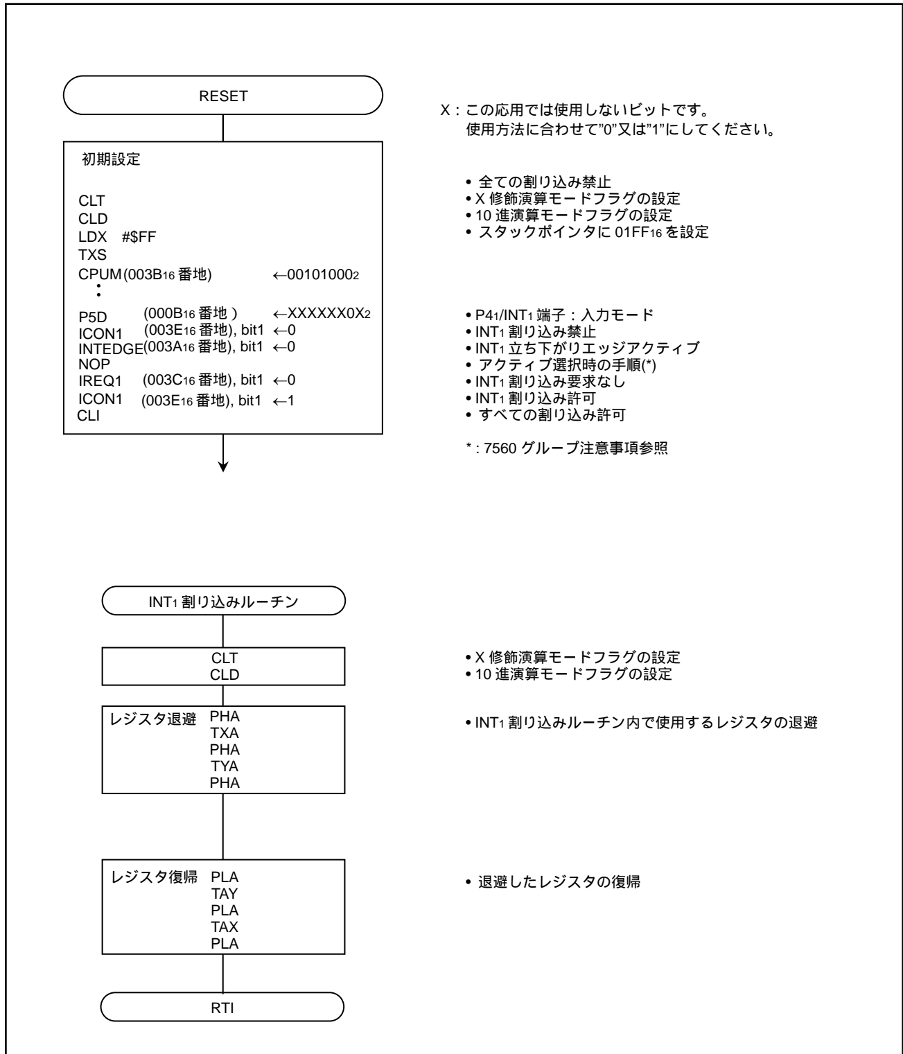
図 3.3 制御手順
