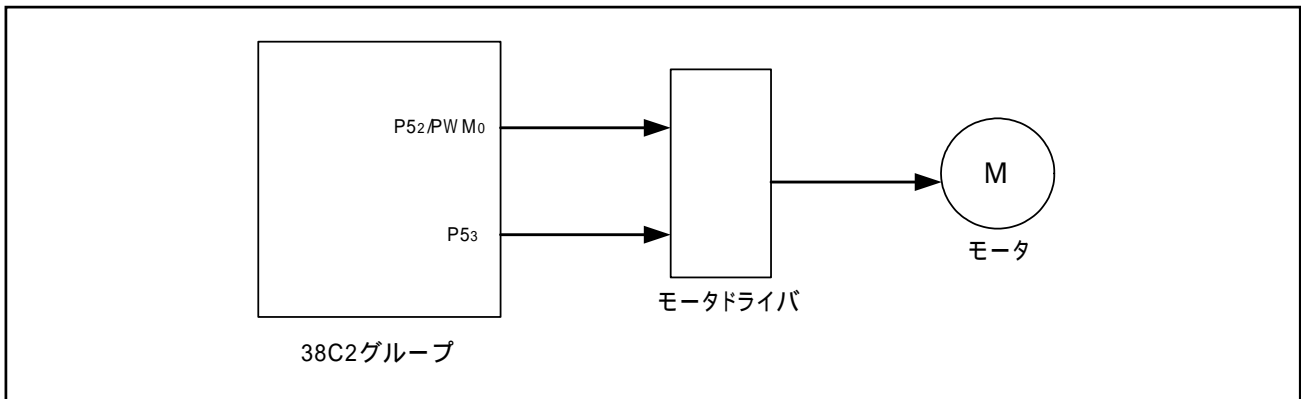
図 3.1 接続図
