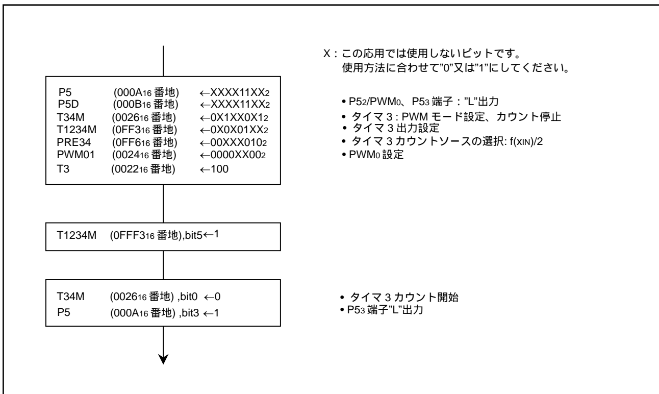
図 3.4 制御手順
