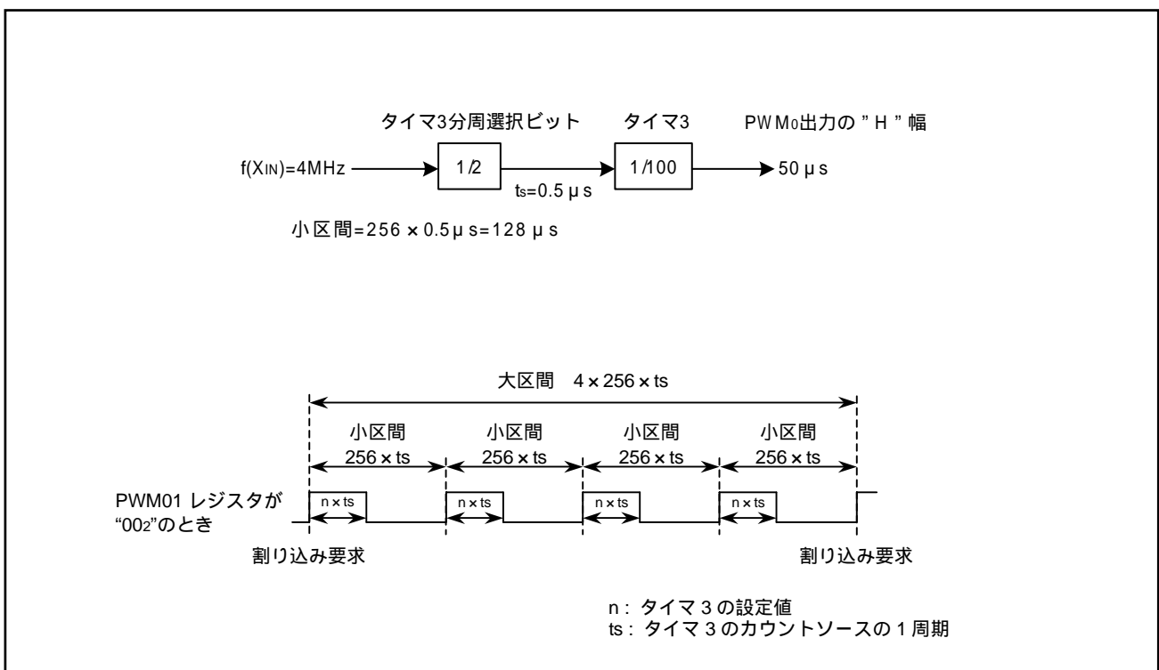
図 3.2 PWM0 の出力波形図
