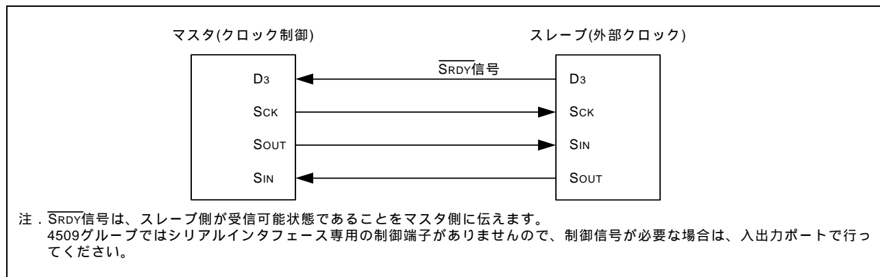
図 4.1 シリアルインタフェース接続例
