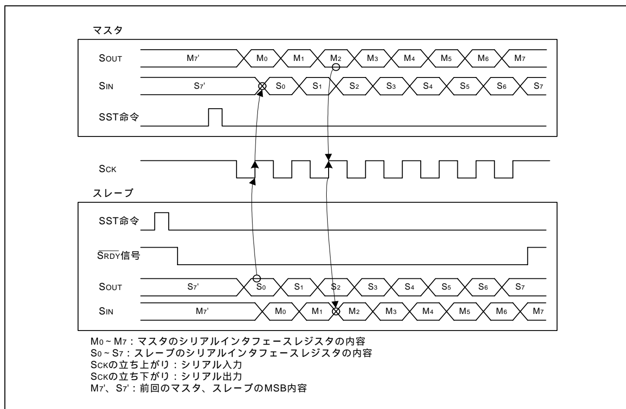
図 4.2 シリアルインタフェース転送タイミング
