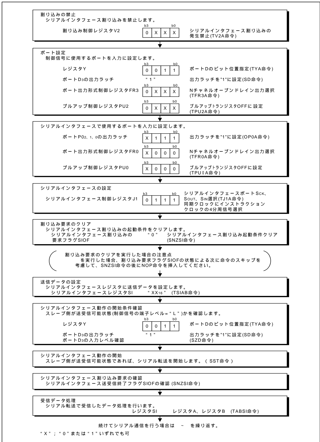
図 5.1 マスタ側シリアルインタフェースの割り込みを使用しない設定例
