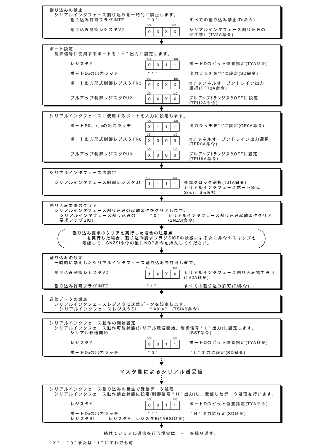
図 5.2 スレーブ側シリアルインタフェースの割り込みを使用する設定例
