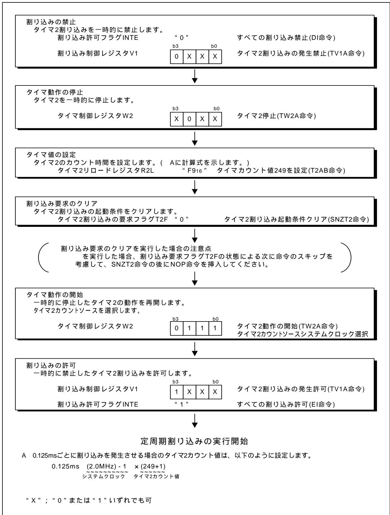
図 4.4 タイマ 2 定周期割り込み設定例
