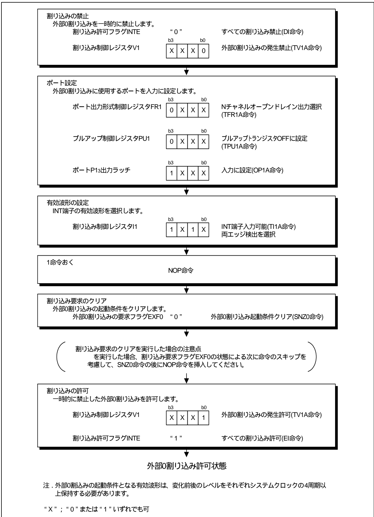
図 4.2 外部 0 割り込み設定例
