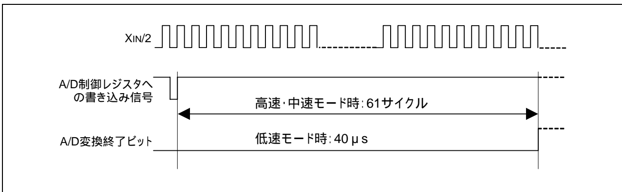
図 3.2 A/D変換タイミングチャート
