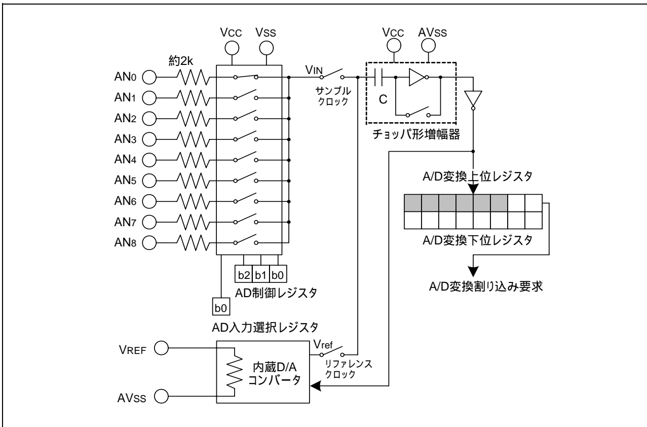
図 3.1 A/Dコンバータ等価回路
