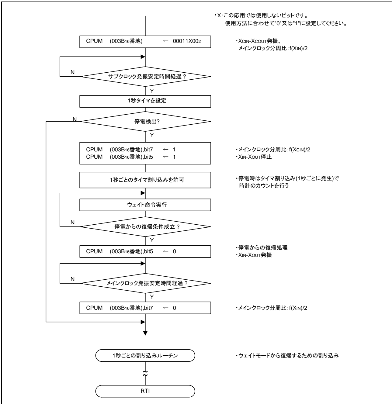
図 3.3 制御手順
