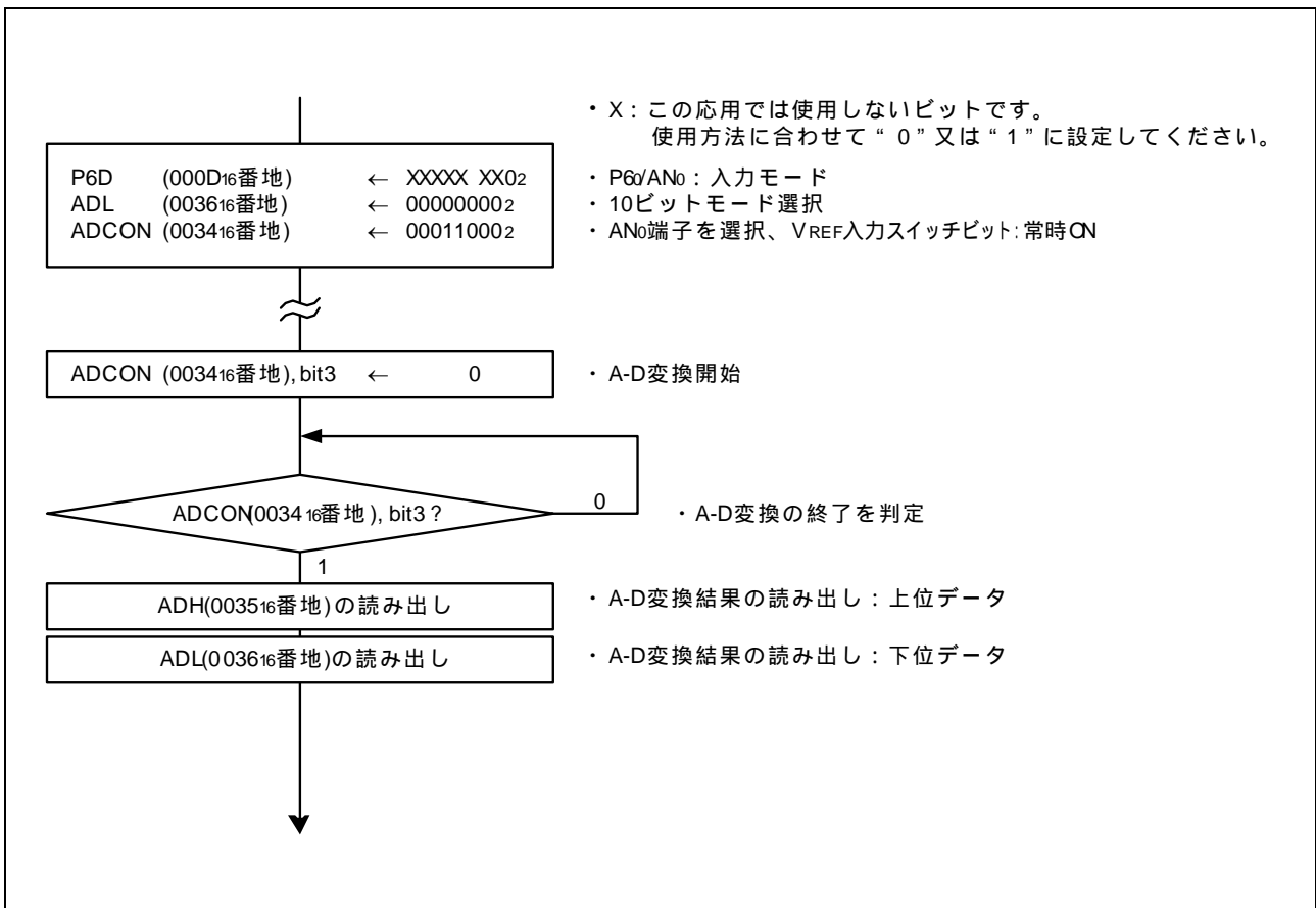
図 3.3 制御手順
