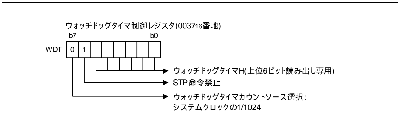
図 3.2 関連レジスタの設定
